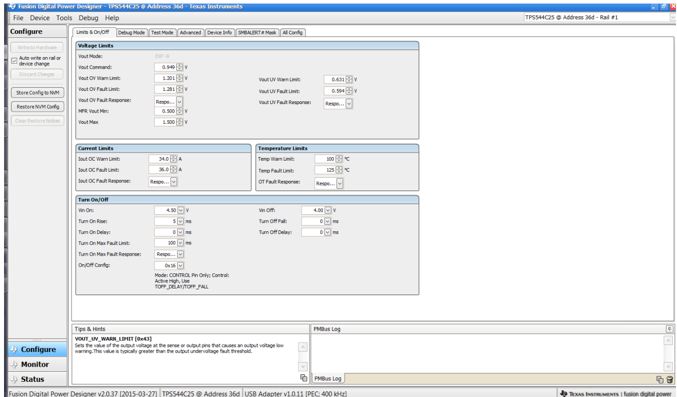
图 58. 使用 Fusion Digital Power Designer 进行器件配置
