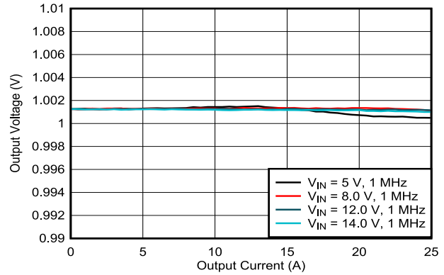
图 7-5. 负载调节
