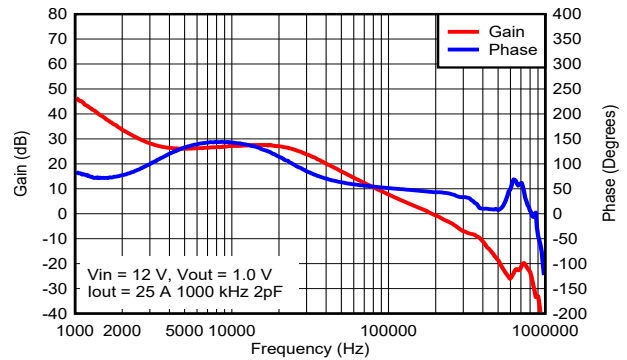
图 7-7. 波特图
