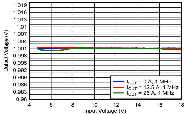
图 7-6. 线性调整率
