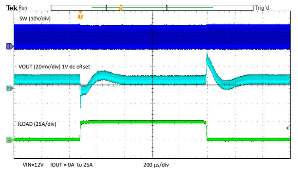
图 7-8. 负载瞬态
