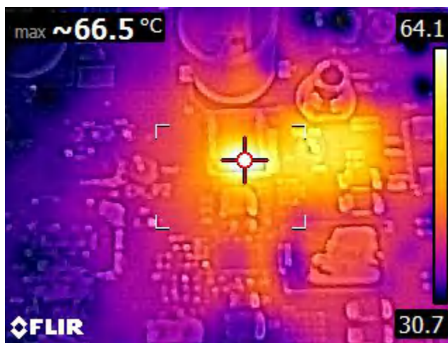
图 7-24. 25°C 环境温度下的热图像
