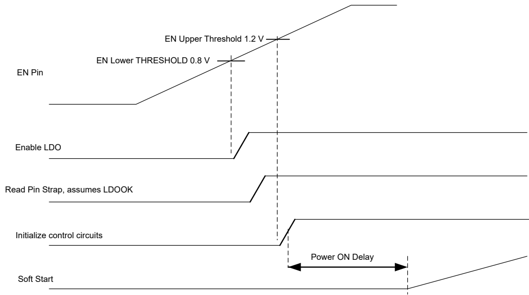
图 6-3. 内部启动序列
