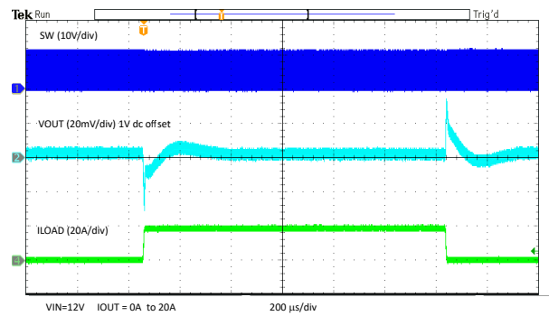
图 7-8. 负载瞬态
