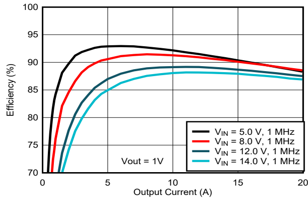
图 7-4. 效率曲线
