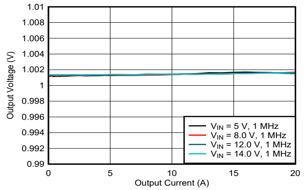
图 7-5. 负载调整率
