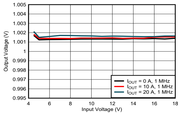
图 7-6. 线路调节
