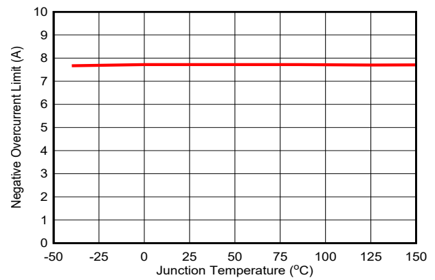
图 5-4. 负过流限制
