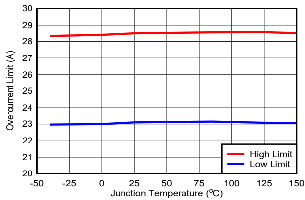
图 5-3. 过流限值
