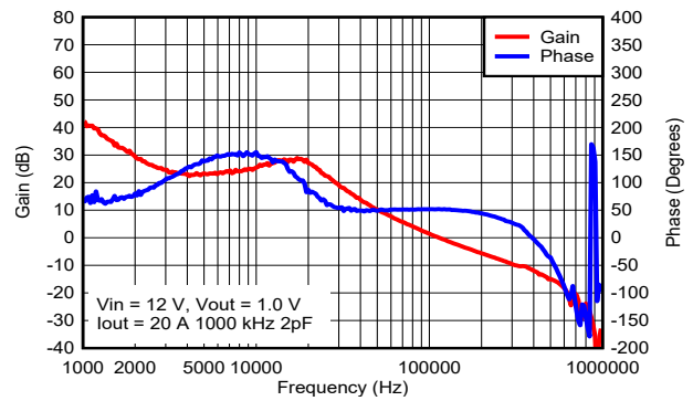
图 7-7. 波特图
