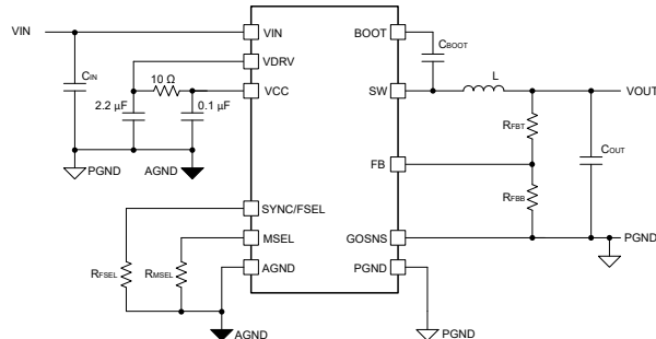
TPS543A26 简化版应用
