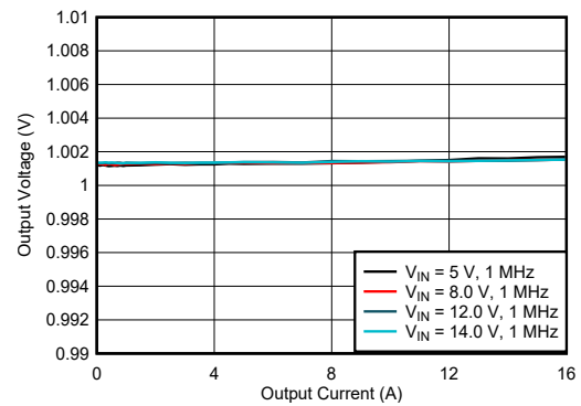
图 7-5. 负载调整率
