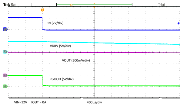
图 7-11. EN 关断
