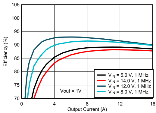
图 7-4. 效率曲线
