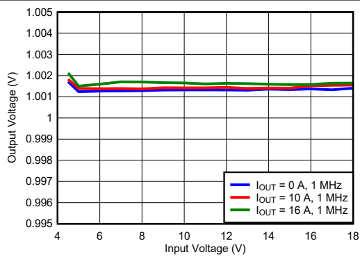
图 7-6. 线路调节
