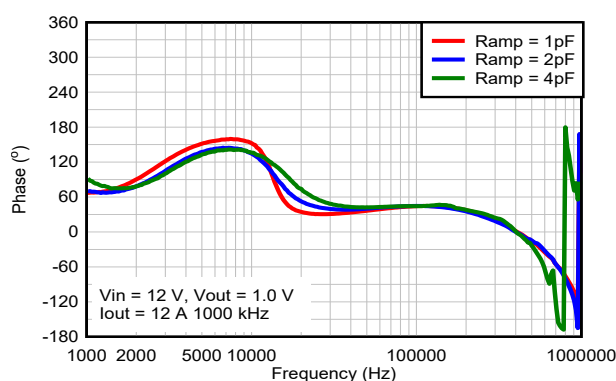
图 6-8. 环路相位与斜坡设置
