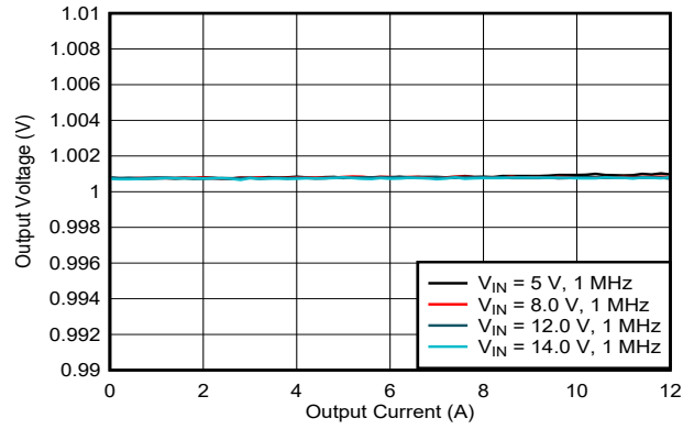
图 7-5. 负载调整率
