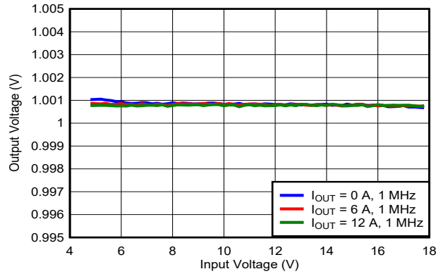
图 7-6. 线路调节
