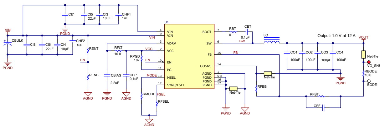
图 7-1. 12V 输入、1.0V 输出、1MHz 原理图
