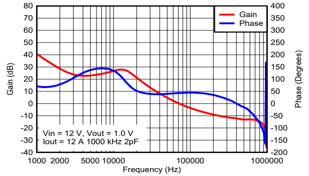
图 7-7. 波特图
