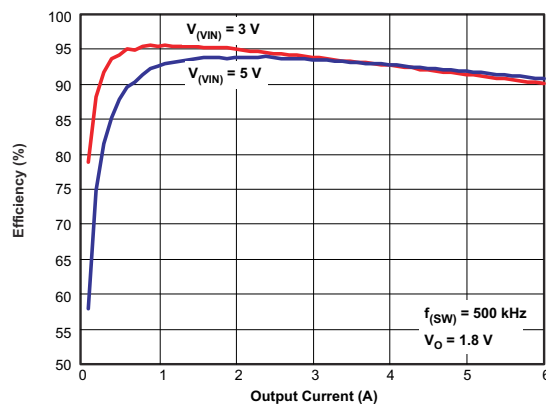
效率曲线
