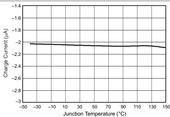
图 6-10. EN Pin Current vs Temperature
