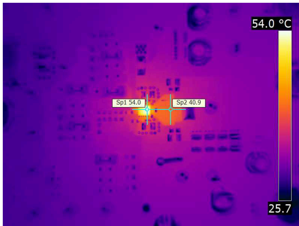
图 10-2. Thermal Image at 25^\circ\text{C} Ambient
