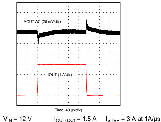
图 8-25. Load Transient
