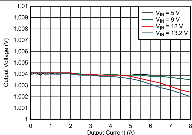
图 8-26. Load Regulation
