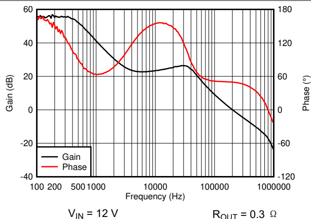
图 8-27. Bode Plot
