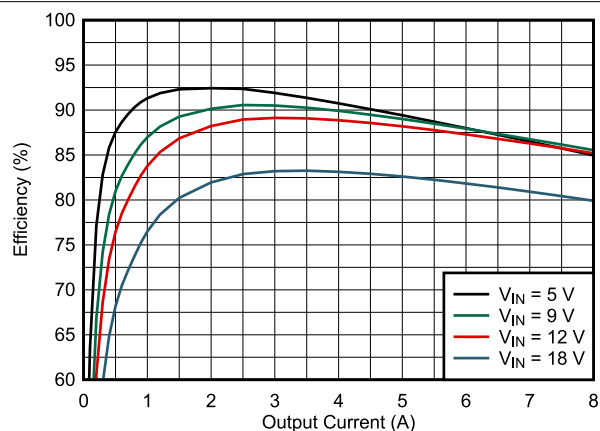
图 8-4. Efficiency
