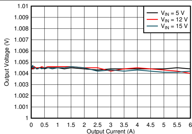
图 8-26. Load Regulation
