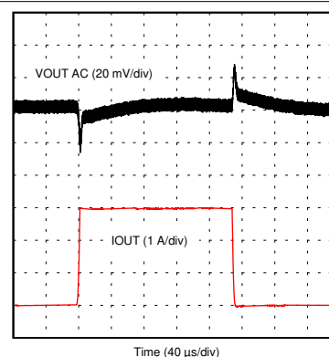
图 8-25. Load Transient
