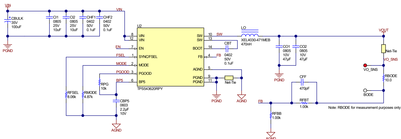
图 8-23. 12-V Input, 1.0-V Output, 1.5-MHz Schematic
