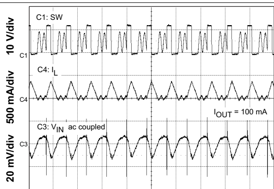
Figure 42. Input Ripple DCM
