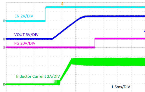
图 7-11. 通过 EN 的启动, I_{OUT} = 5A
