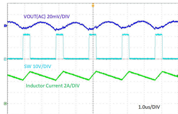
图 7-13. 稳态, I_{OUT} = 5A
