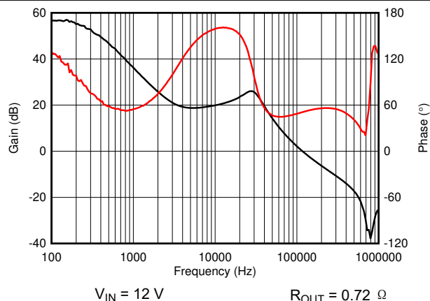
图 8-25. Bode Plot
