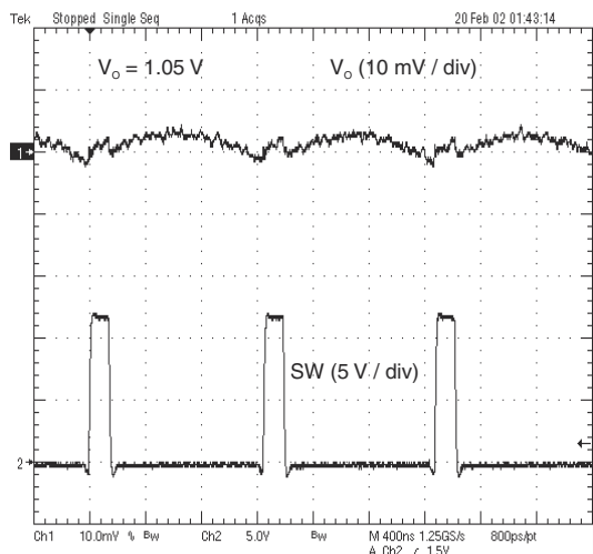
图 8-6. Voltage Ripple at Output
