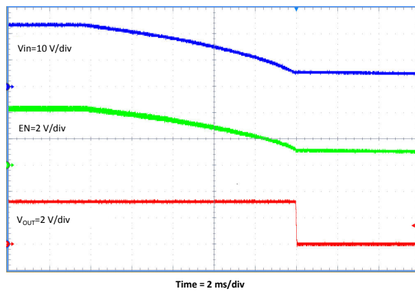
图 8-13. 相对于 VIN 的关断
