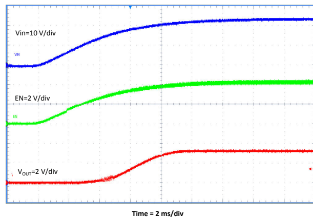
图 8-12. 相对于 VIN 的启动
