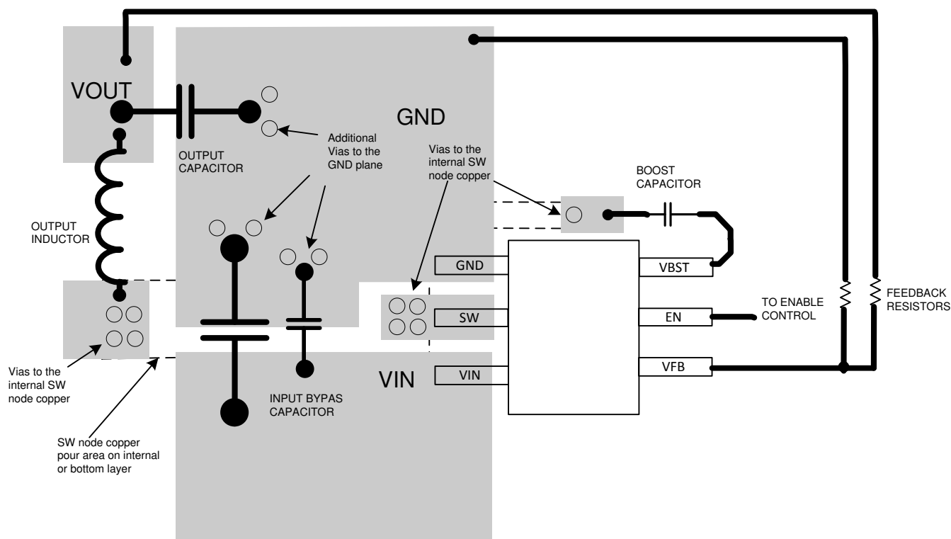
图 10-1. 电路板布局
