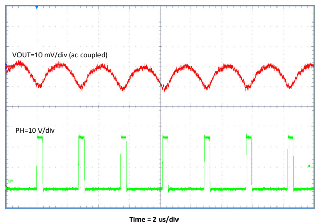
图 8-6. 输出电压纹波
