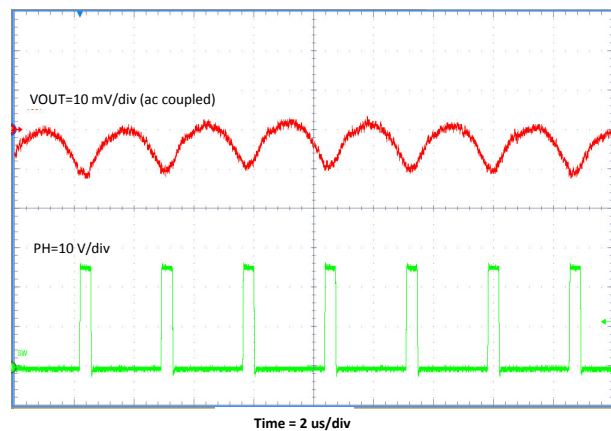
图 8-8. 输出电压纹波
