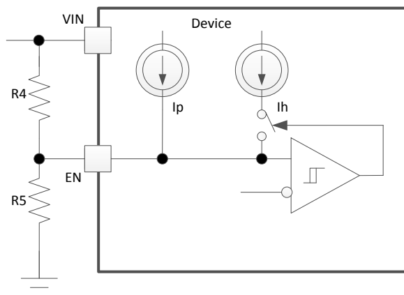
图 7-1. 可调节 VIN 欠压锁定
