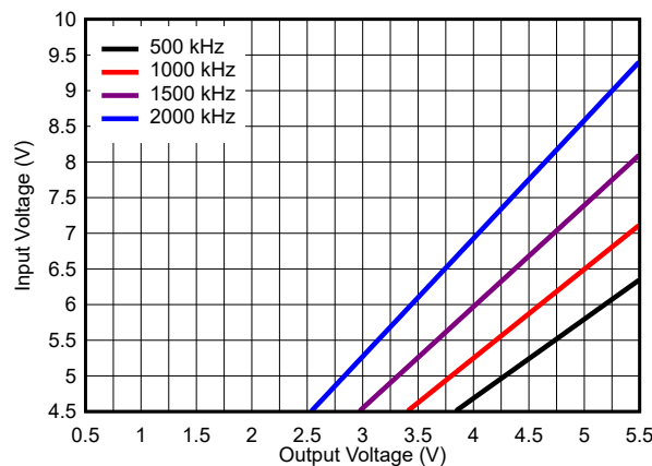
图 7-2. Minimum Input Voltage
