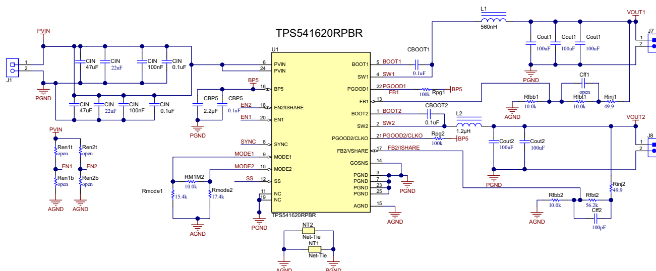
图 8-1. 12-V 输入, 1.0-V 和 3.3-V 双输出调节器应用示意图
