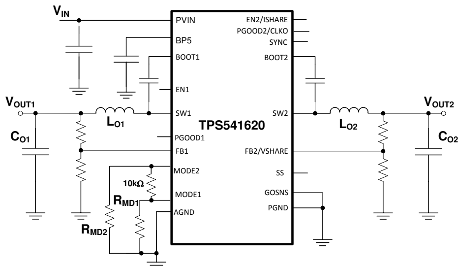
简化原理图 (双路输出)
