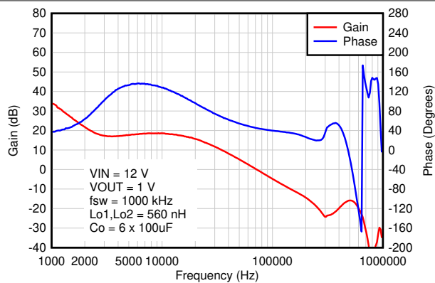
图 8-37. Bode Plot
