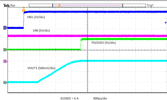
图 8-15. Power Up with EN 1
