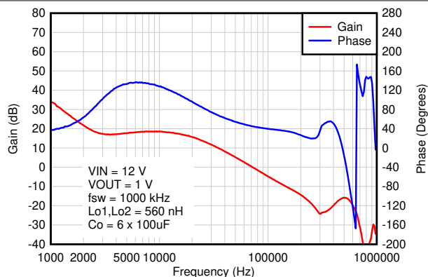
图 8-37. Bode Plot
