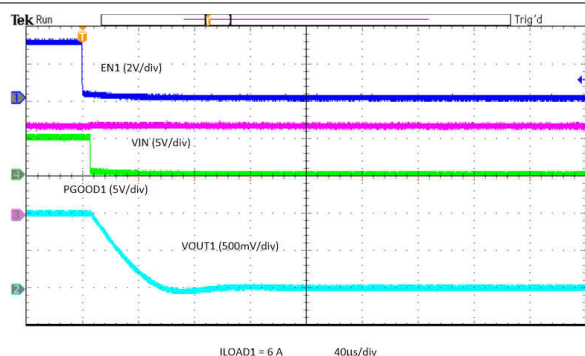
图 8-17. Power Down with EN 1
