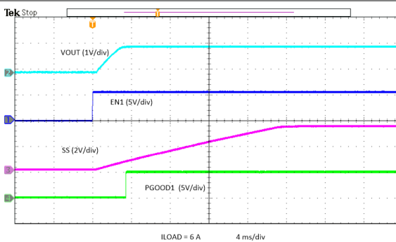
图 8-39. Power Up with EN
