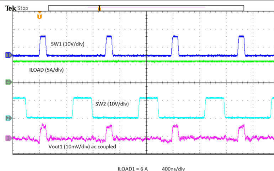
图 8-28. V_{OUT1} Output Ripple - 6-A Load
