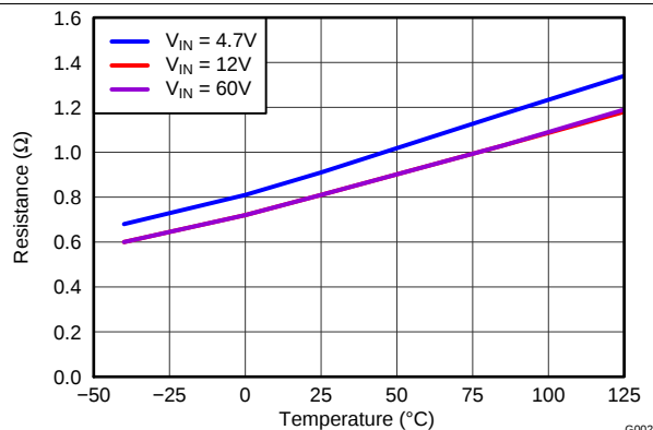
Figure 2. 低侧 R_{DS(on)} 与温度间的关系
