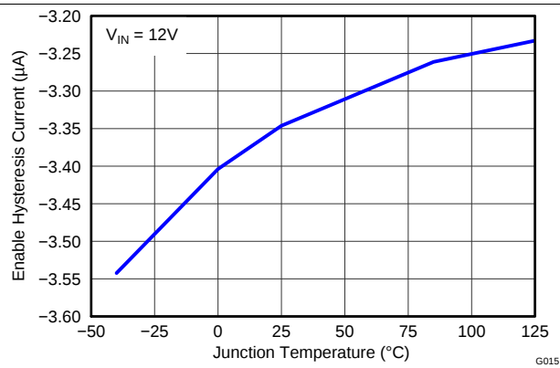
Figure 9. 使能引脚迟滞电流与温度间的关系
