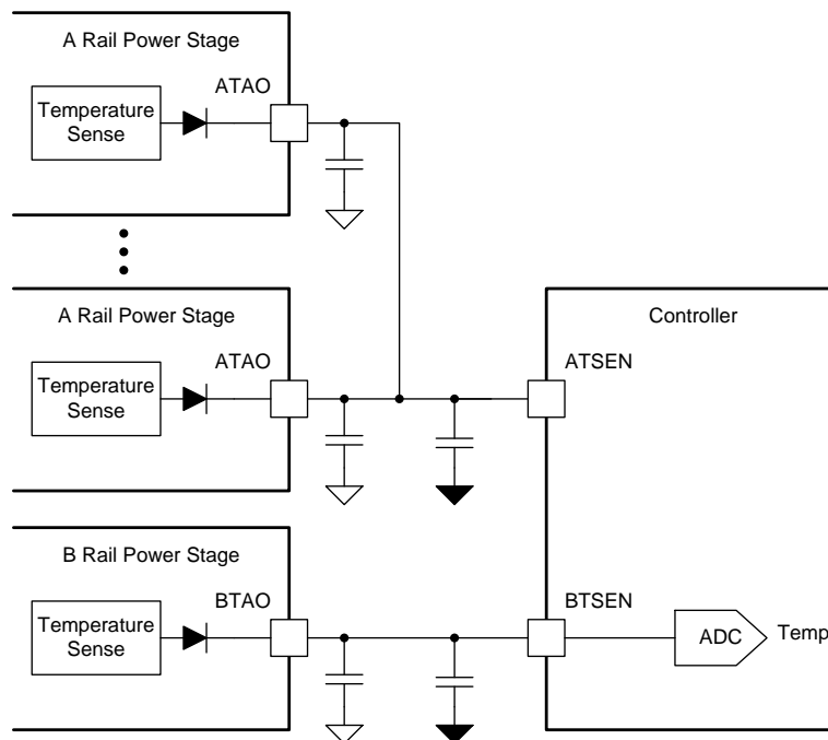
图 10. Temperature Sense
