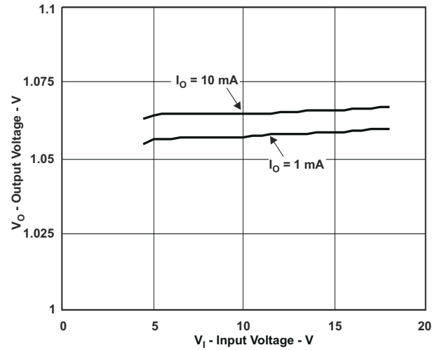
图 8-3. 1.05-V Output Voltage vs. Input Voltage
