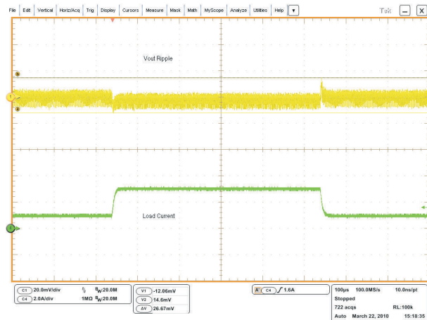
图 8-4. 1.05-V, 0-A to 3-A Load Transient Response
