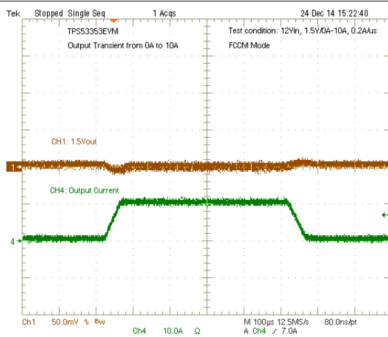
图 8-9. Output Transient with FCCM Mode
