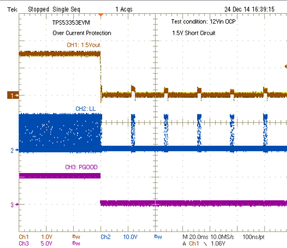
图 8-12. Output Short-Circuit Protection
