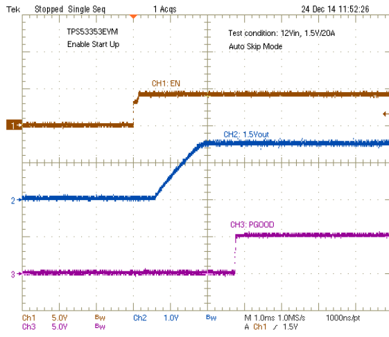
图 8-5. Enable Turnon
