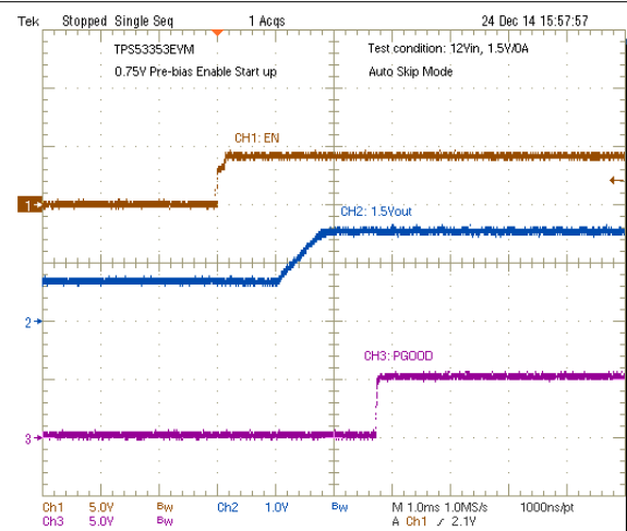
图 8-10. Output 0.75-V Prebias Turnon
