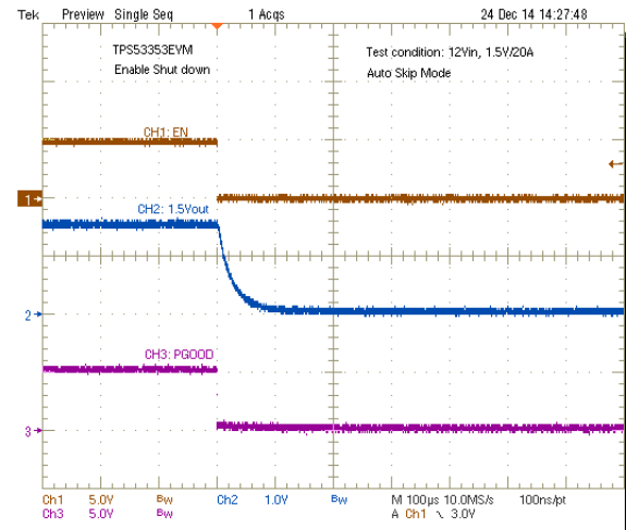
图 8-6. Enable Turnoff
