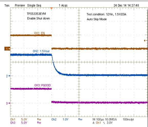
图 8-3. Enable Turnoff
