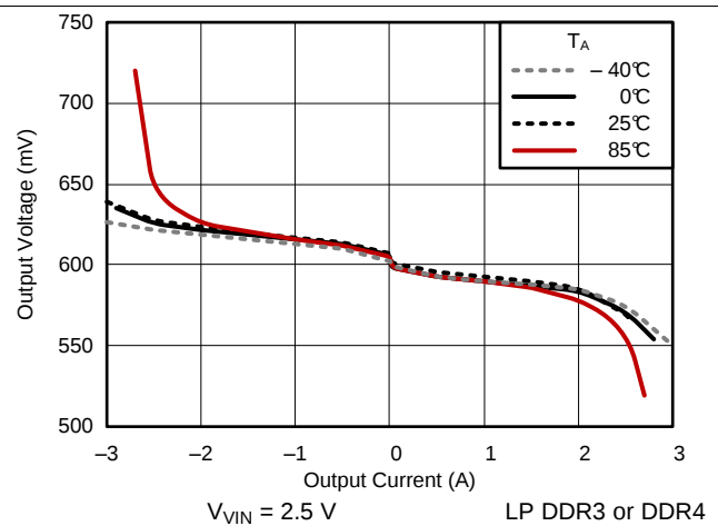
图 10. Load Regulation
