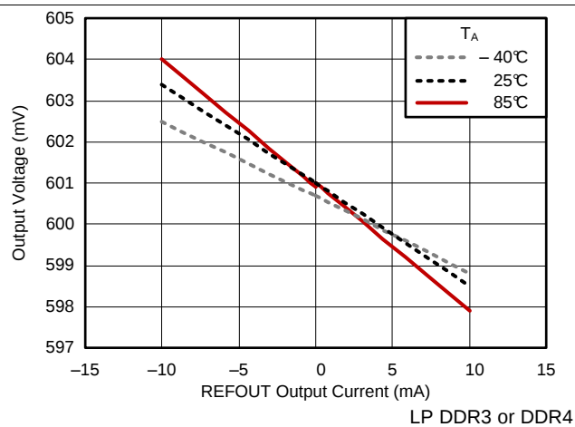
图 13. REFOUT Load Regulation
