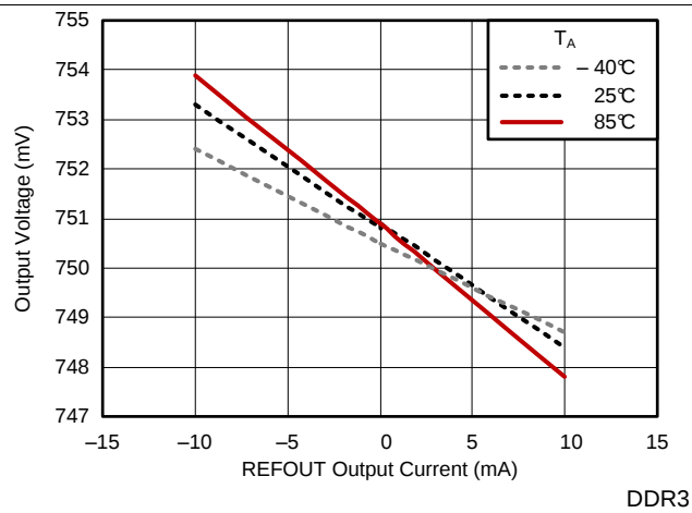
图 11. REFOUT Load Regulation
