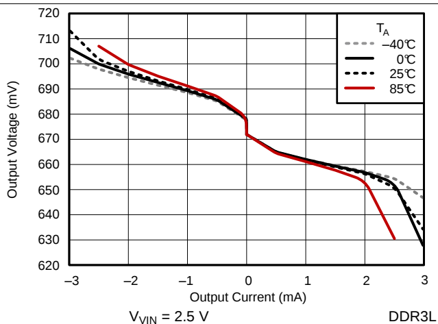
图 9. Load Regulation
