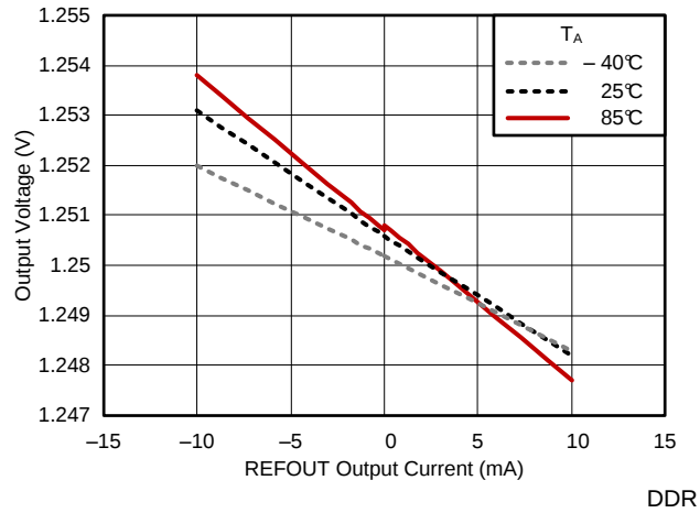
图 11. REFOUT Load Regulation
