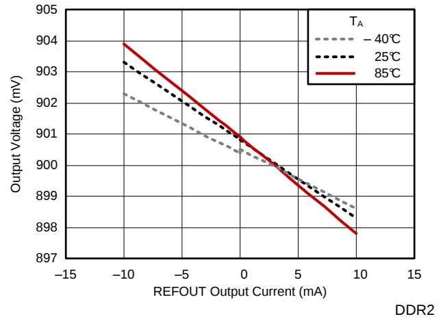
图 12. REFOUT Load Regulation
