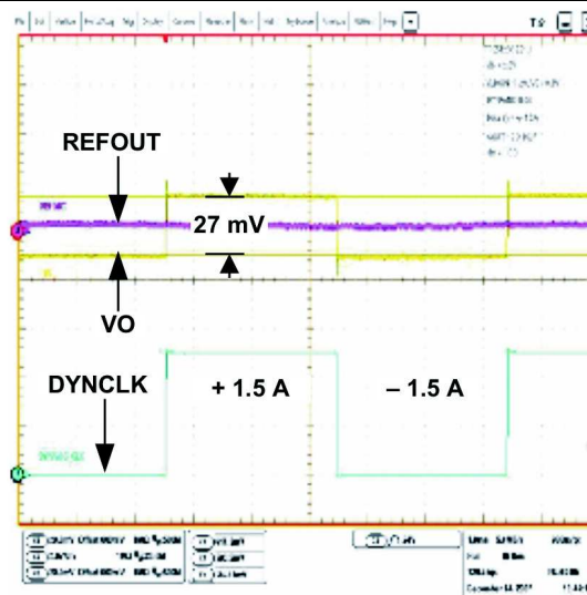
图 25. Transient Waveform
