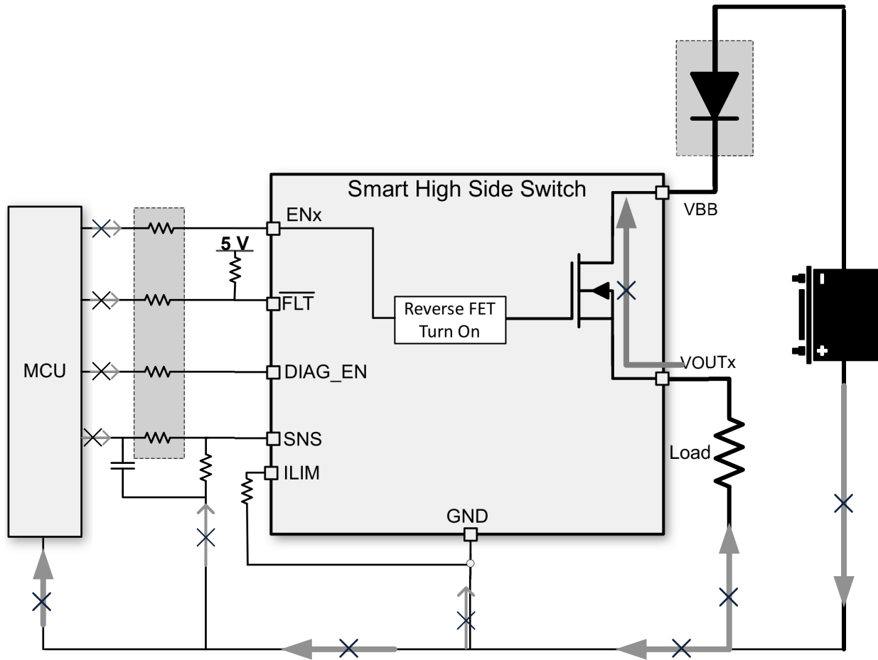
图 7-21. 采用阻断二极管实现反向保护
