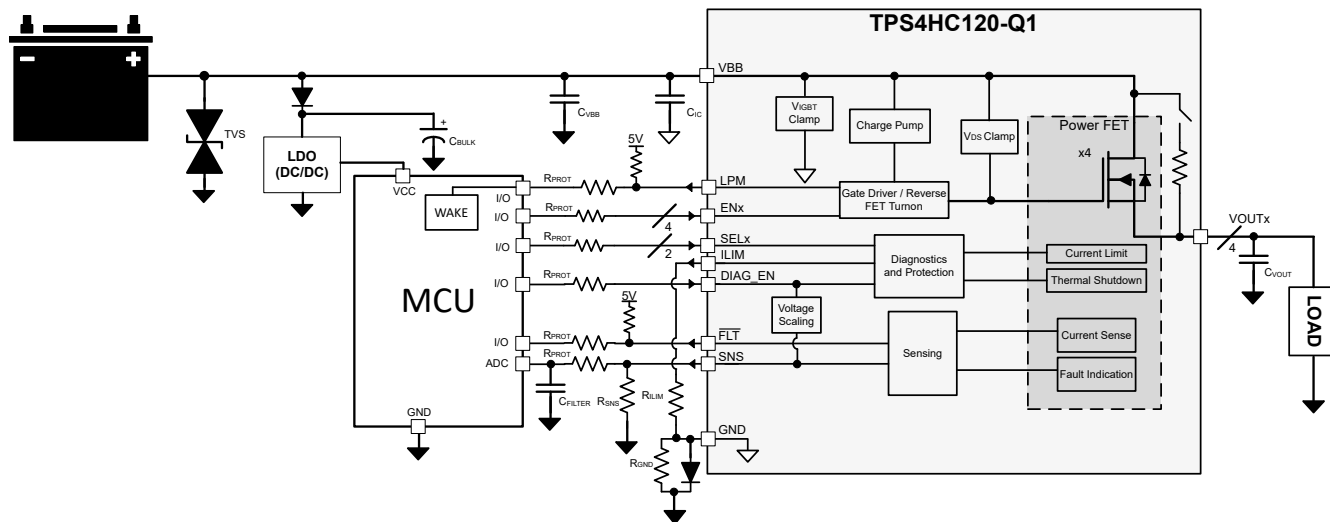
图 8-1. 典型应用图
