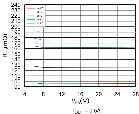
图 6-5. 不同温度条件下 R_{ON} 与 V_{BB} 间的关系
