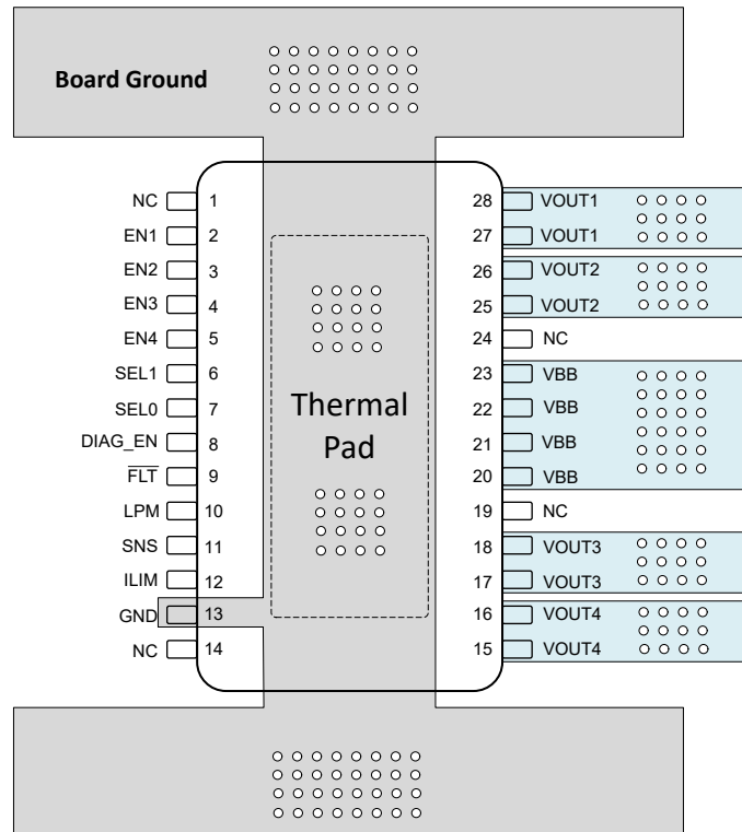
图 8-4. 无接地网络的布局示例
