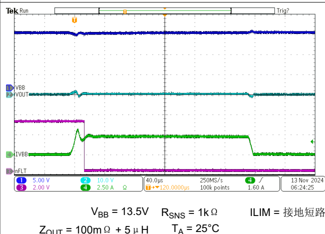
图 6-18. ILIM 接地短路时的永久短路行为
