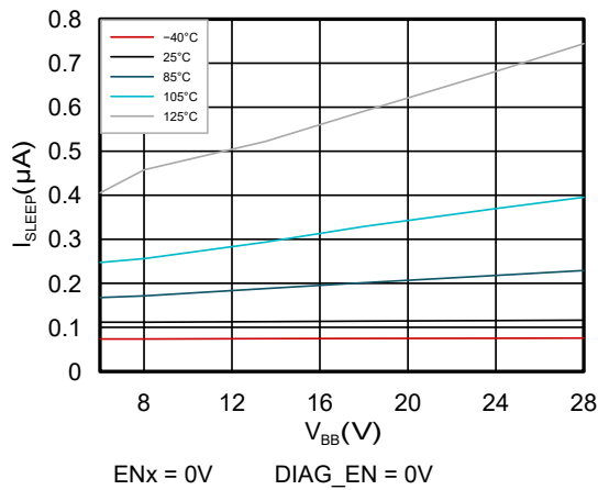
图 6-3. 不同温度条件下 I_{SLEEP} 与 V_{BB} 间的关系
