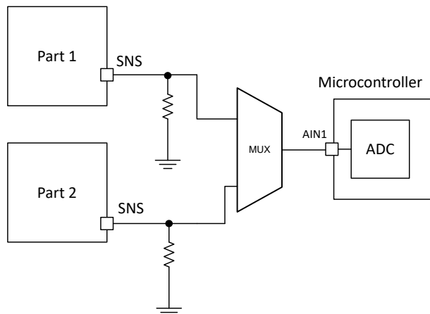
图 7-14. 跨多个器件共享 SNS 方法 2
