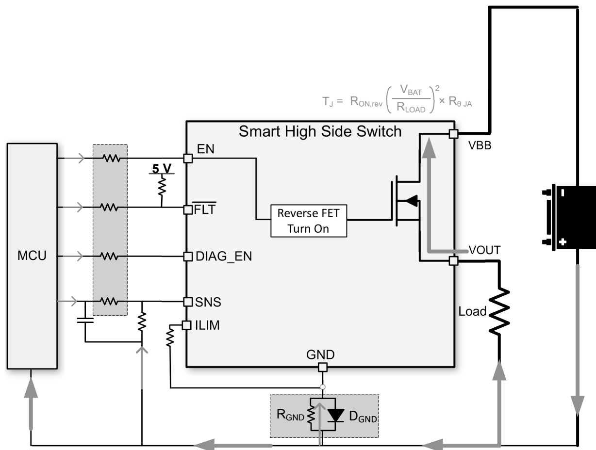
图 7-22. 通过接地网络实现反向保护
