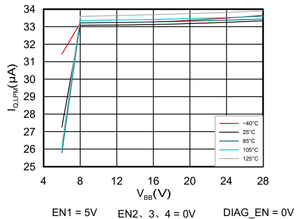
图 6-6. 启用 1 个通道时, 不同温度条件下 I_{Q,LPM} 与 V_{BB} 间的关系
