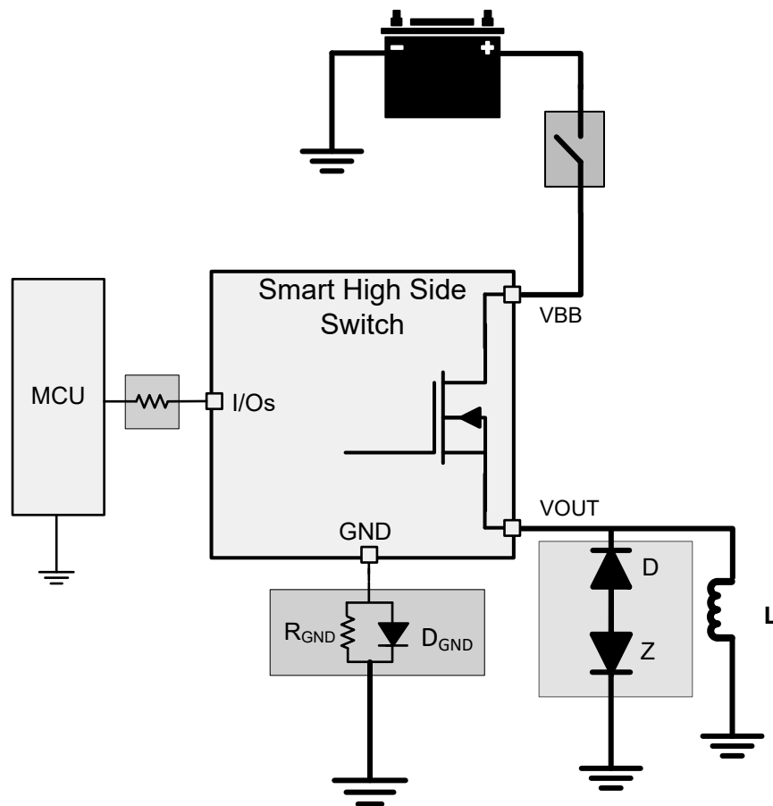
图 7-20. 电池丢失
