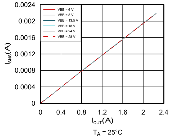
图 6-2. V_{BB} 电压范围内 I_{SNS} 与 I_{OUT} 间的关系
