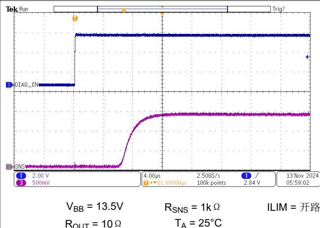
图 6-16. DIAG_EN 导通时的 SNS 引脚电压
