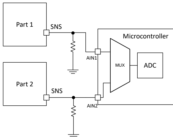
图 7-13. 跨多个器件共享 SNS 方法 1
