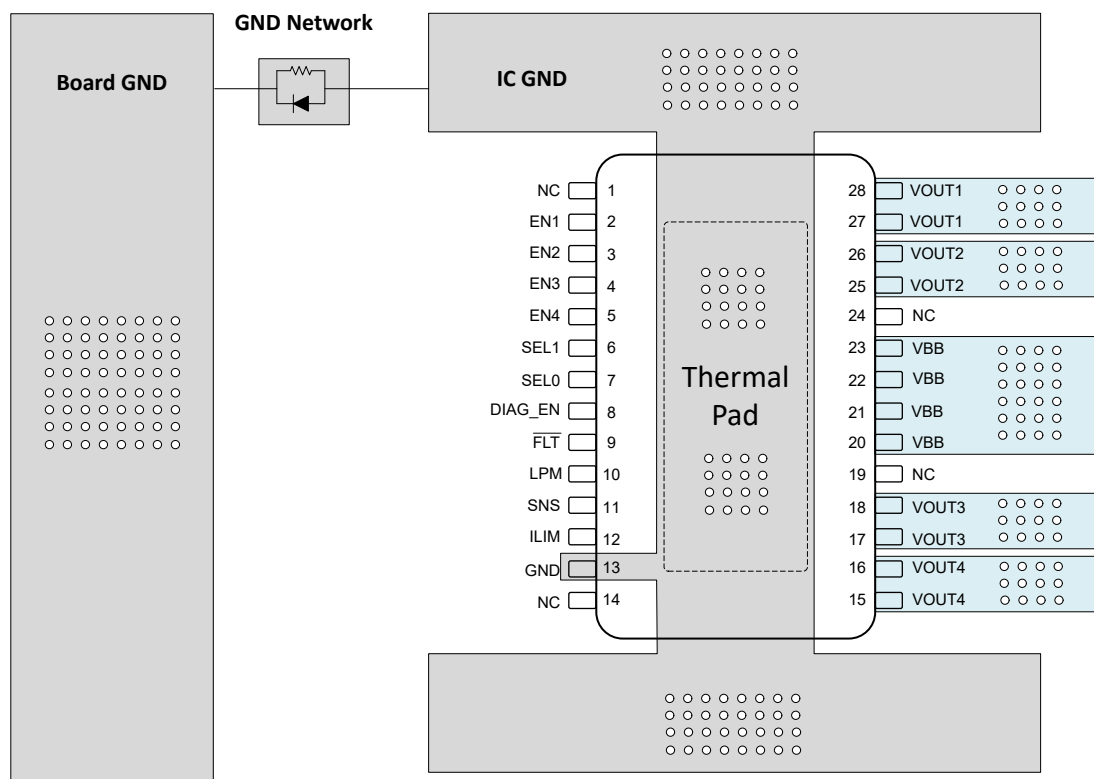
图 8-5. 有接地网络的布局示例
