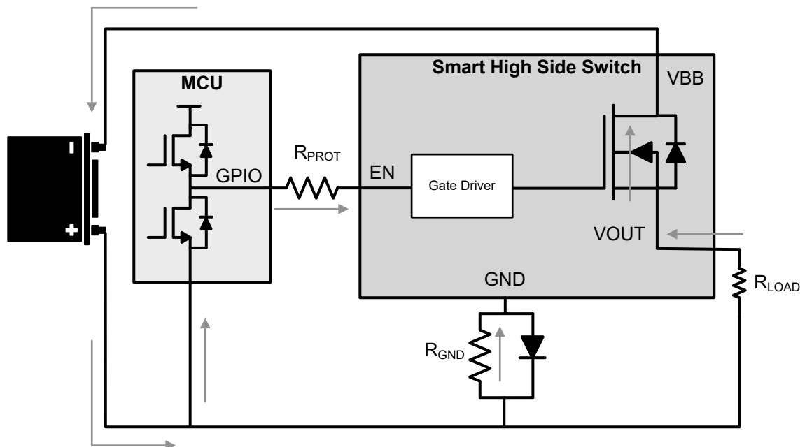
图 7-16. 电池反向电路
