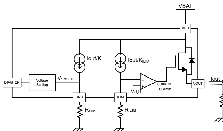
图 7-6. 电流检测和电流限制方框图
