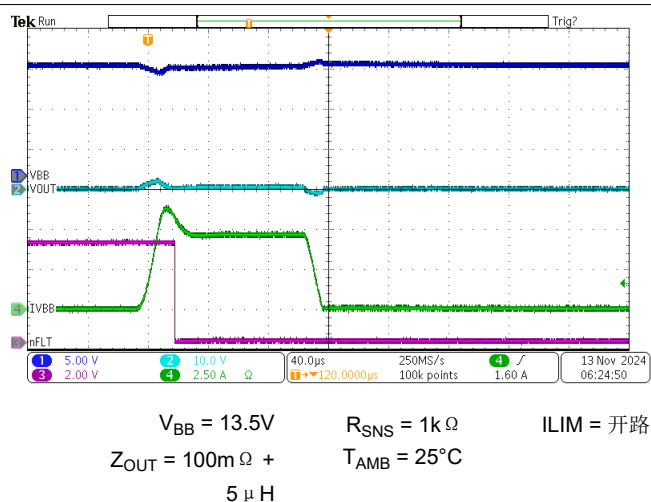
图 6-17. ILIM 开路时的永久短路行为
