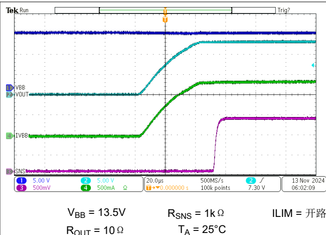
图 6-14. 开关导通
