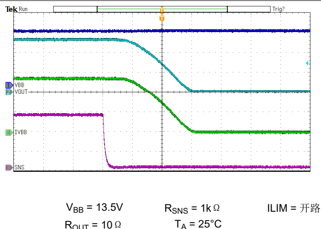
图 6-15. 开关关断
