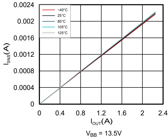
图 6-1. 不同温度条件下 I_{SNS} 与 I_{OUT} 间的关系
