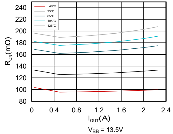
图 6-4. 不同温度条件下 R_{ON} 与 I_{OUT} 间的关系
