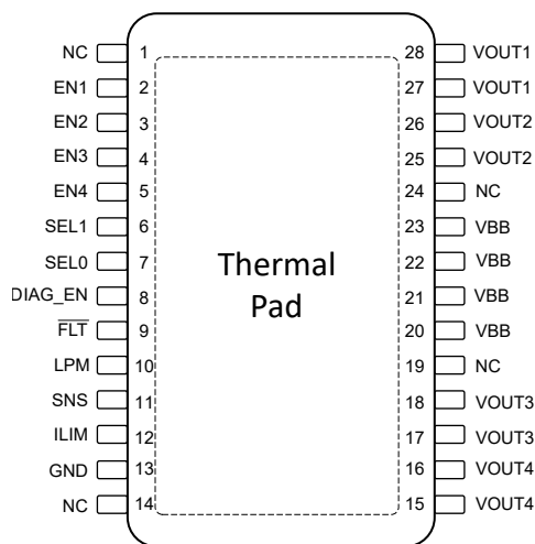
图 5-1. DGQ 封装，28 引脚 HVVSOP (俯视图)
