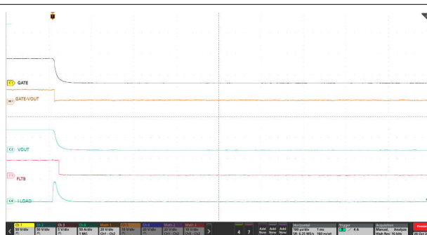
图 9-7. TPS4816-Q1 的输出短路响应
