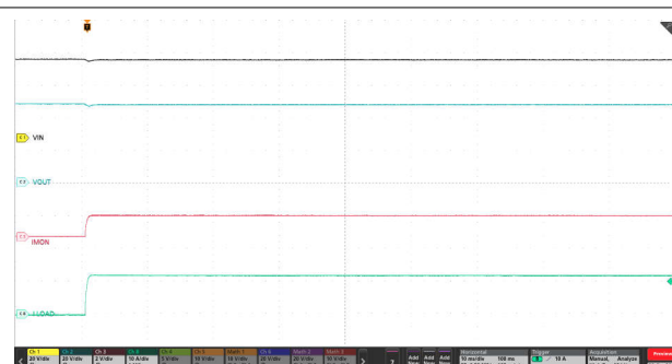
图 9-8. TPS4816-Q1 电流监测输出 (IMON) 瞬态响应
