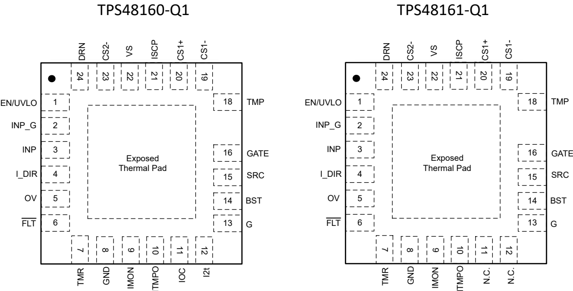
图 5-1. RGE 封装，23 引脚 VQFN ( 俯视图 )
