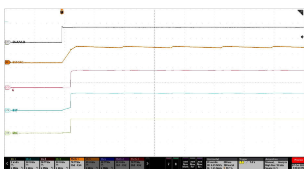
图 9-2. 旁路路径的启动曲线 ( INP_G = 高电平, VIN = 48V, 无负载, C BST = 470nF )
