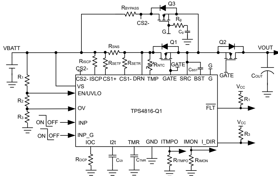
图 9-1. 使用 TPS4816-Q1 驱动电容负载
