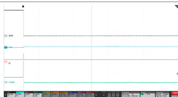
图 9-6. TPS4816-Q1 在 I²t 过流故障下的闭锁响应
