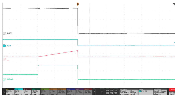
图 9-3. 6A 至 16A 负载阶跃下 TPS4816-Q1 EVM 基于 I²t 的过流响应
