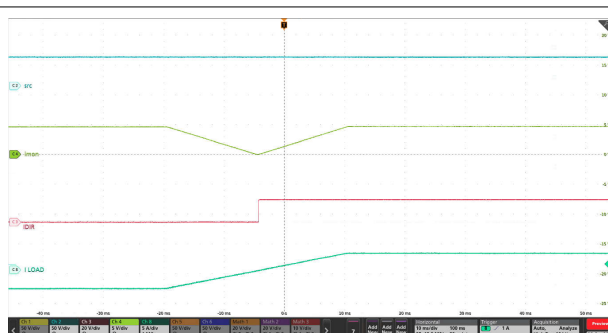
图 9-9. TPS4816-Q1 双向电流监测输出 ( IMON、I_DIR ) 瞬态响应
