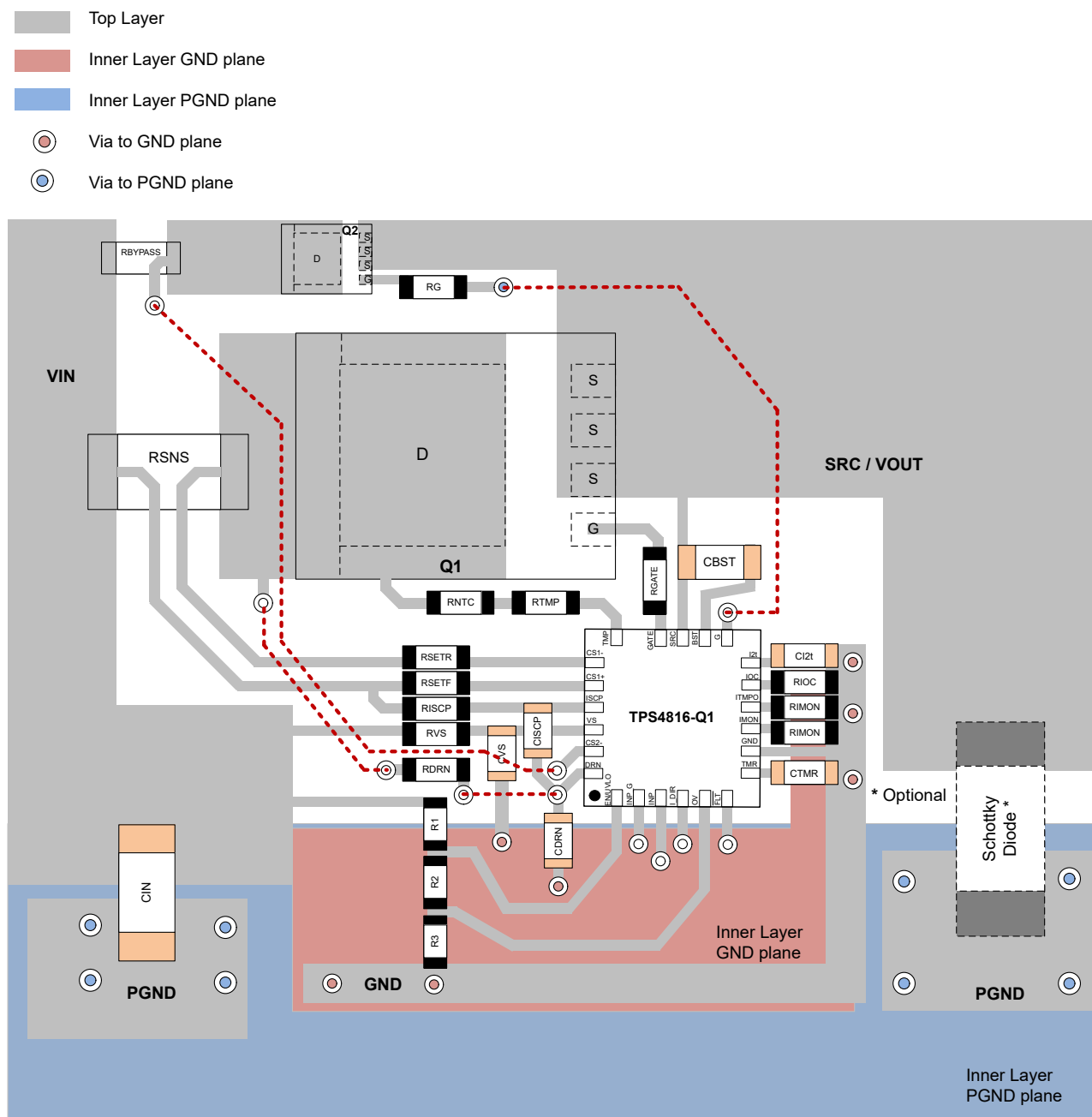
图 9-14. TPS4816-Q1 的典型 PCB 布局布线示例
