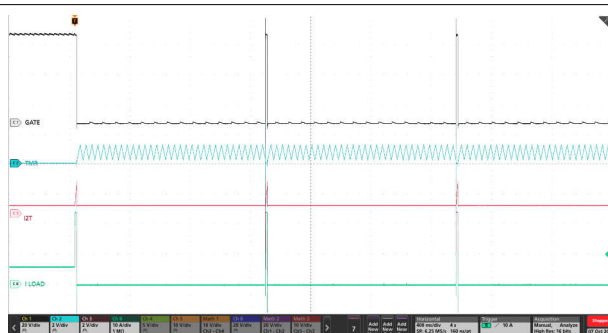
图 9-5. TPS4816-Q1 在 I²t 过流故障下的自动重试响应
