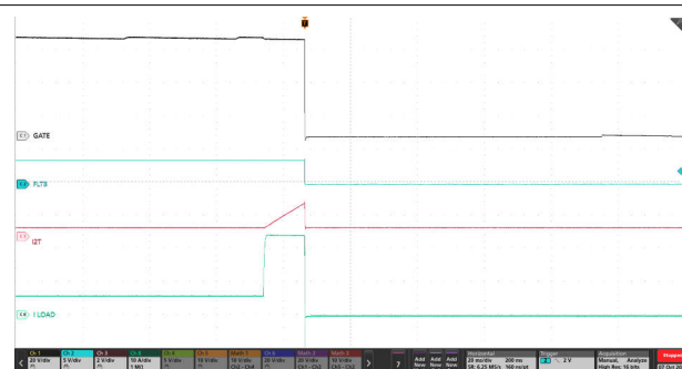
图 9-4. 6A 至 23A 负载阶跃下 TPS4816-Q1 EVM 基于 I²t 的过流响应
