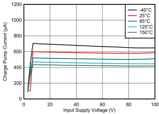
图 6-3. 电荷泵电流与电源电压间的关系
