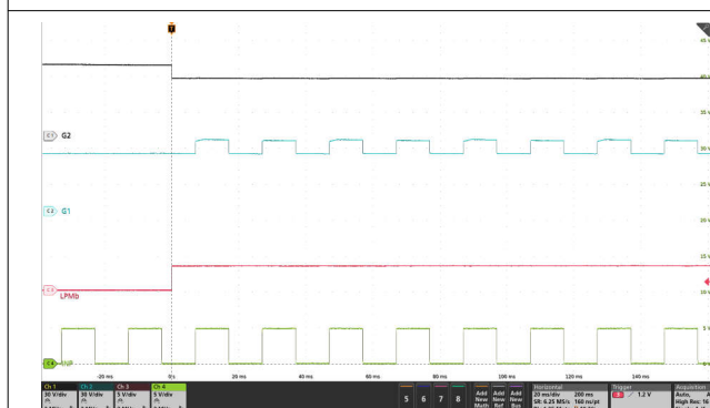
图 8-6. 当 \overline{\text{LPM}} = 低电平到高电平时，INP 获得对 G1 的控制 (VIN = 48V，无负载)
