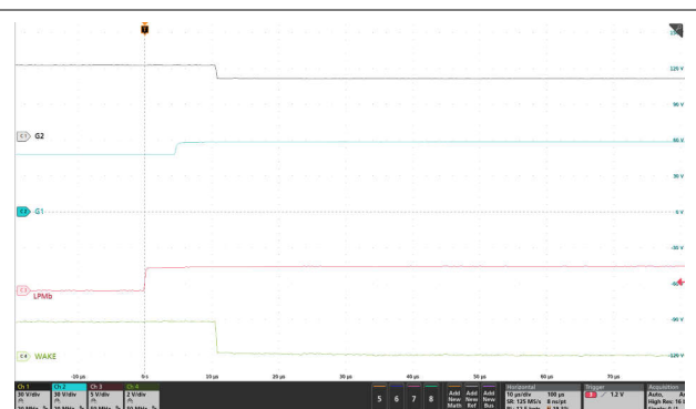
图 8-5. 从 LPM 到工作模式的状态转换 ( \overline{\text{LPM}} = 低电平到高电平，VIN = 48V，无负载)
