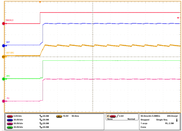
图 8-3. INP = GND、 C_{BST} = 470\text{nF} 时自举电压的启动曲线
