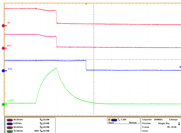
图 8-9. TPS48000-Q1 器件在 15A 短路保护设置且 TMR = 开路的情况下的输出短路响应
