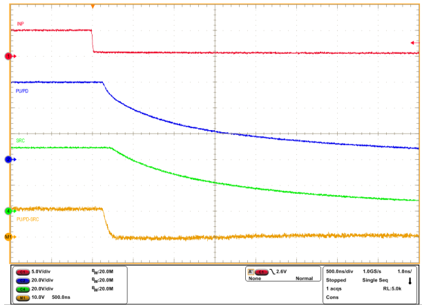
图 8-5. INP 由高电平到低电平且 C_{BST} = 470\text{nF} 时 TPS48000-Q1 的关断响应
