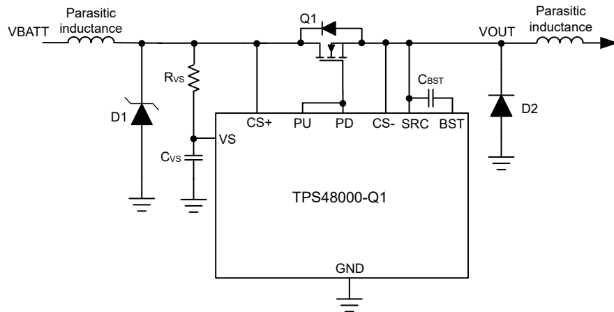
图 8-12. 采用可选保护元件的 TPS48000-Q1 电路实施方案
