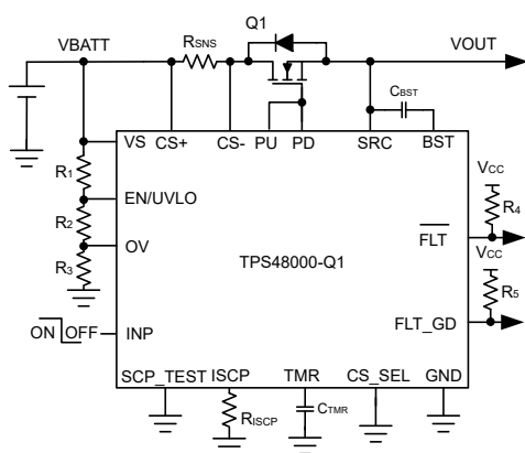
图 7-5. 具有基于外部检测电阻 RSNS 的高电平端电流检测功能的 TPS48000-Q1 应用电路
