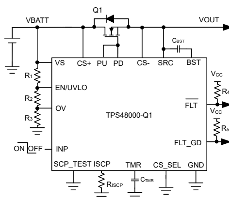
图 7-6. 具有基于 MOSFET R_{DS(on)} 电流检测功能的 TPS48000-Q1 应用电路
