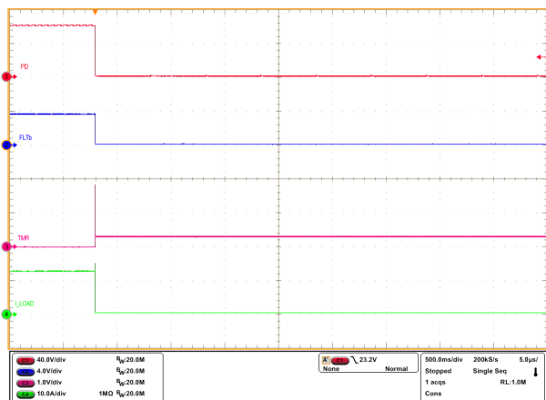
图 8-8. TPS48000-Q1 针对过流故障的闭锁响应
