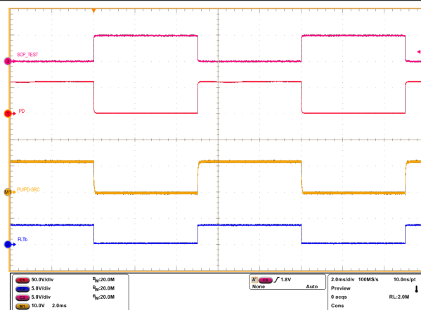
图 8-11. TPS48000-Q1 的短路保护诊断测试响应
