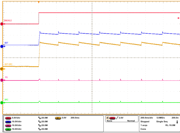
图 8-2. INP = GND、 C_{BST} = 470\text{nF} 时自举电压的启动曲线
