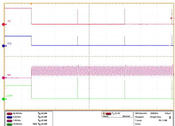
图 8-7. TPS48000-Q1 针对过流故障的自动重试响应
