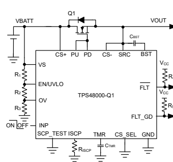
具有高侧 VDS 检测和低侧电流检测的配置
