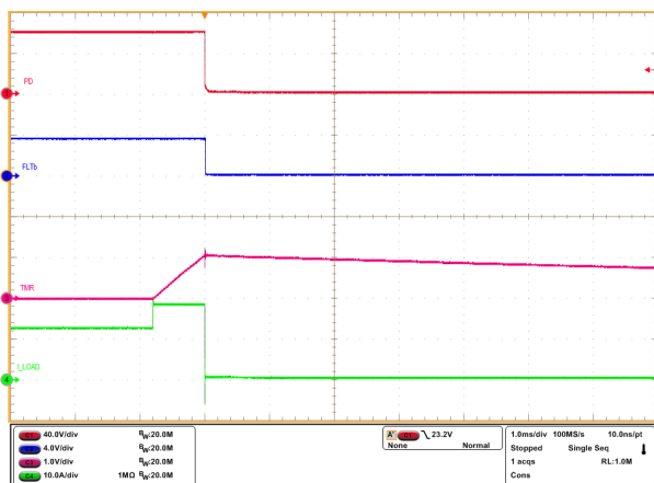
图 8-6. TPS48000-Q1 在 15A 短路保护设置且 t_{sc} = 1\text{ms} 的情况下针对 12A 至 18A 负载阶跃的过流响应
