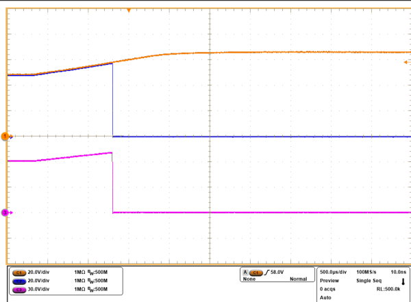
图 8-10. TPS48000-Q1 在 58V 电平下的过压截止响应
