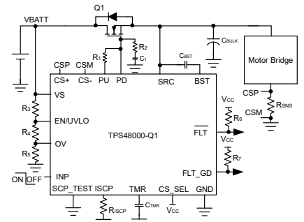
具有高侧 VDS 检测和低侧电流检测的配置
