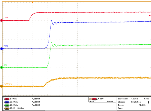
图 8-4. INP 由低电平到高电平且 C_{BST} = 470\text{nF} 时 TPS48000-Q1 的导通响应
