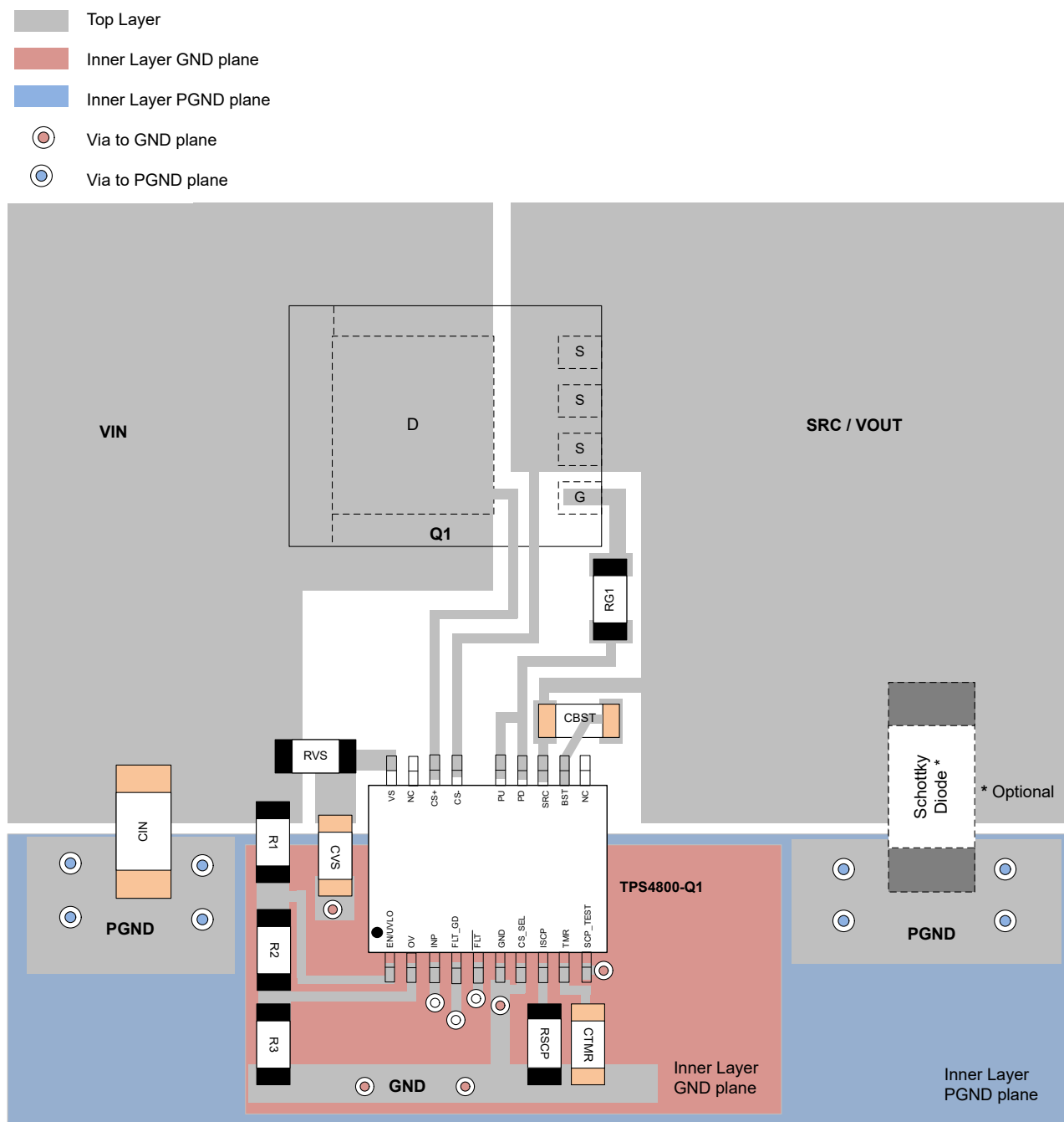
图 8-13. 具有基于 VDS 电流检测的 TPS4800-Q1 典型 PCB 布局示例
