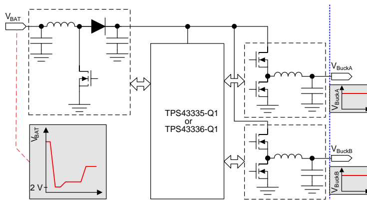
典型应用图
