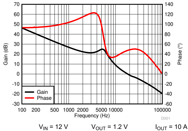
图 9-4. Bode Plot
