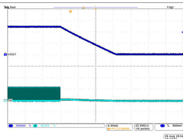
图 9-9. Shutdown from CNTL
