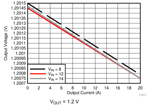
图 9-3. Line Regulation
