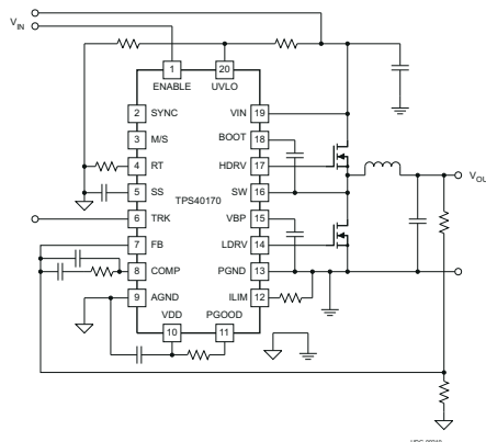
简化版原理图
