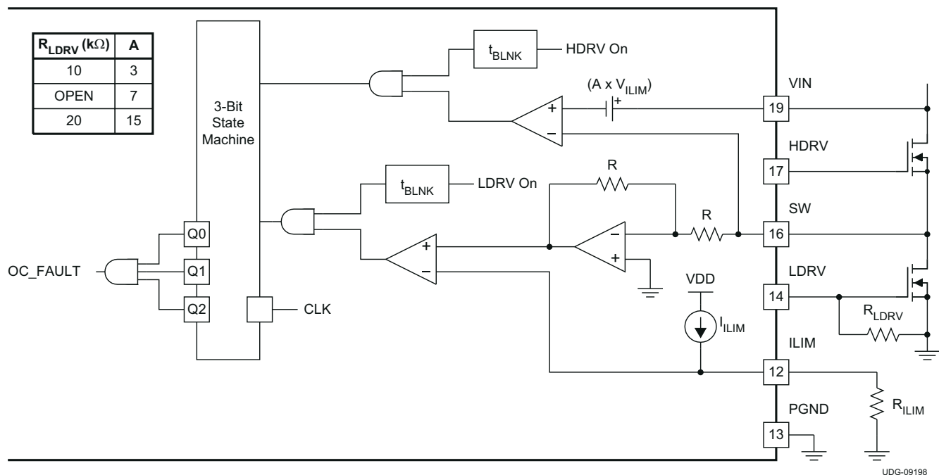
图 6-3. OCP 和 SCP 保护功能块 diagram
