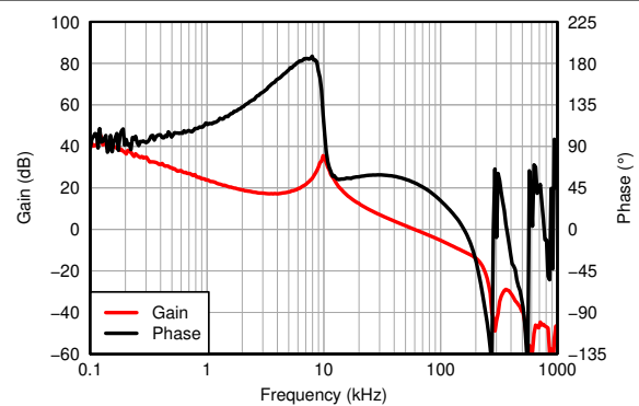
图 7-3. Loop Response
