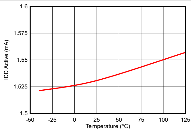
图 6-2. 有效输入电流与温度间的关系
