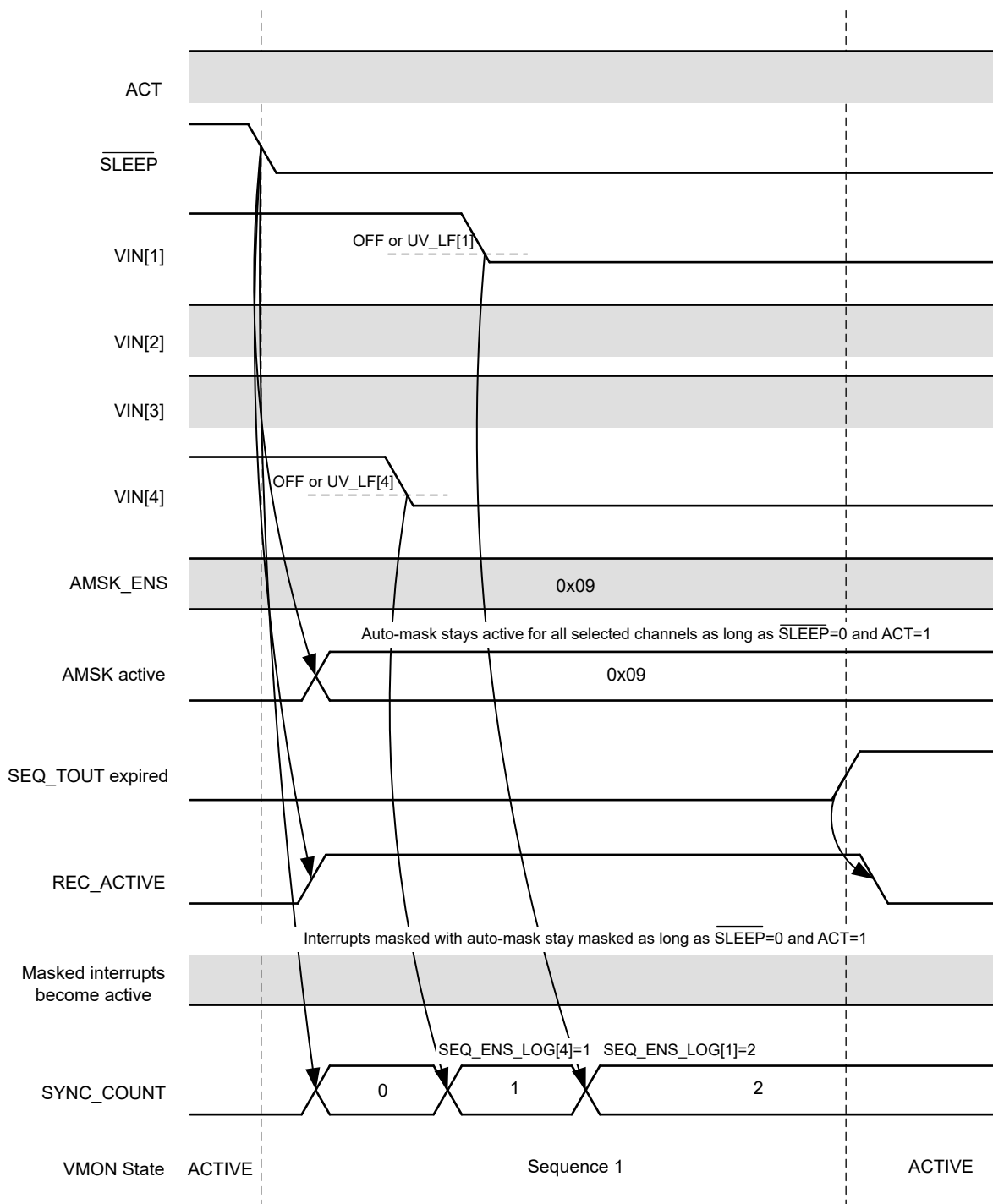
图 7-15. SLEEP 1→0 转换
