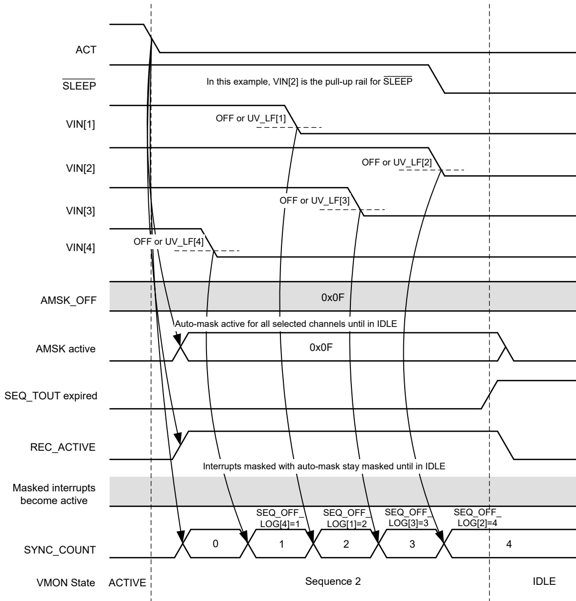
图 7-17. ACT 1→0 转换
