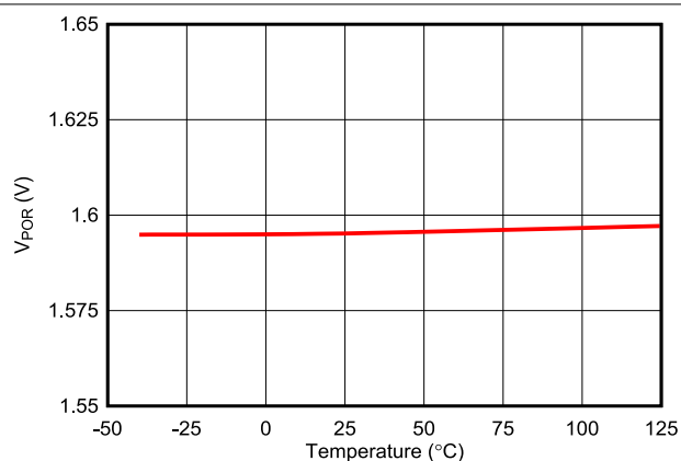
图 6-6. 上电复位电压与温度间的关系
