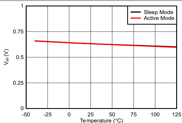
图 6-4. 高电平输入电压与温度间的关系
