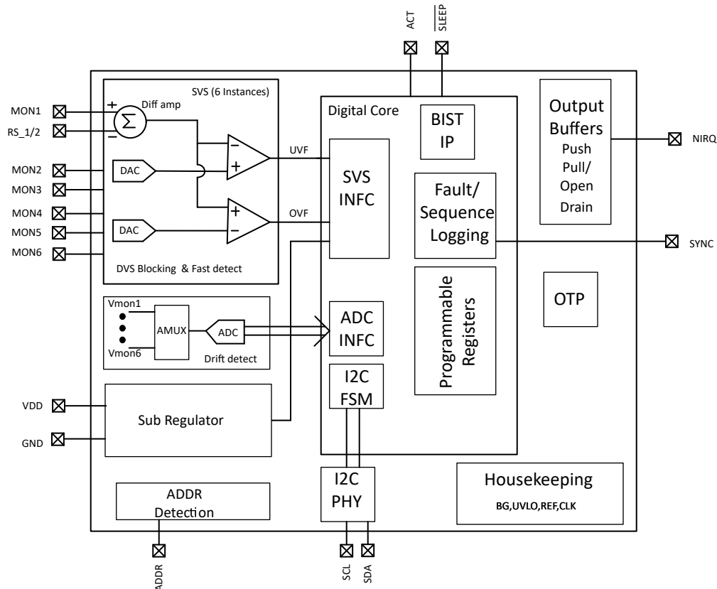
图 7-1. TPS389006-Q1 方框图
