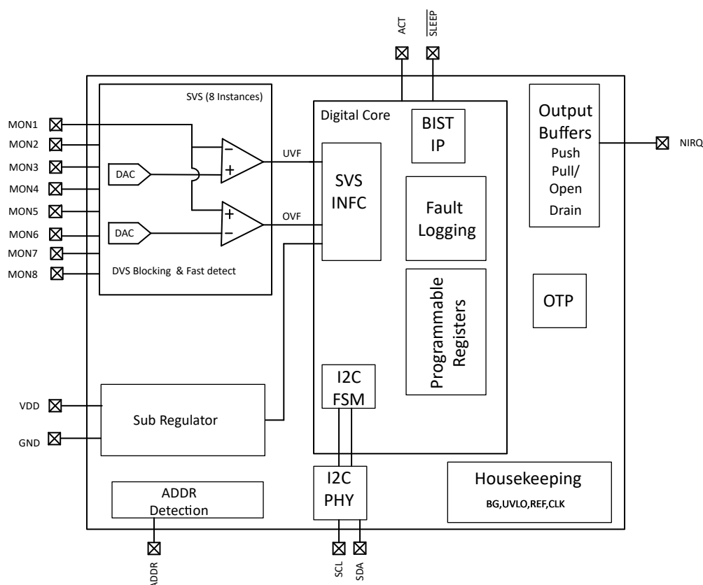
图 7-1. TPS38800-Q1 方框图
