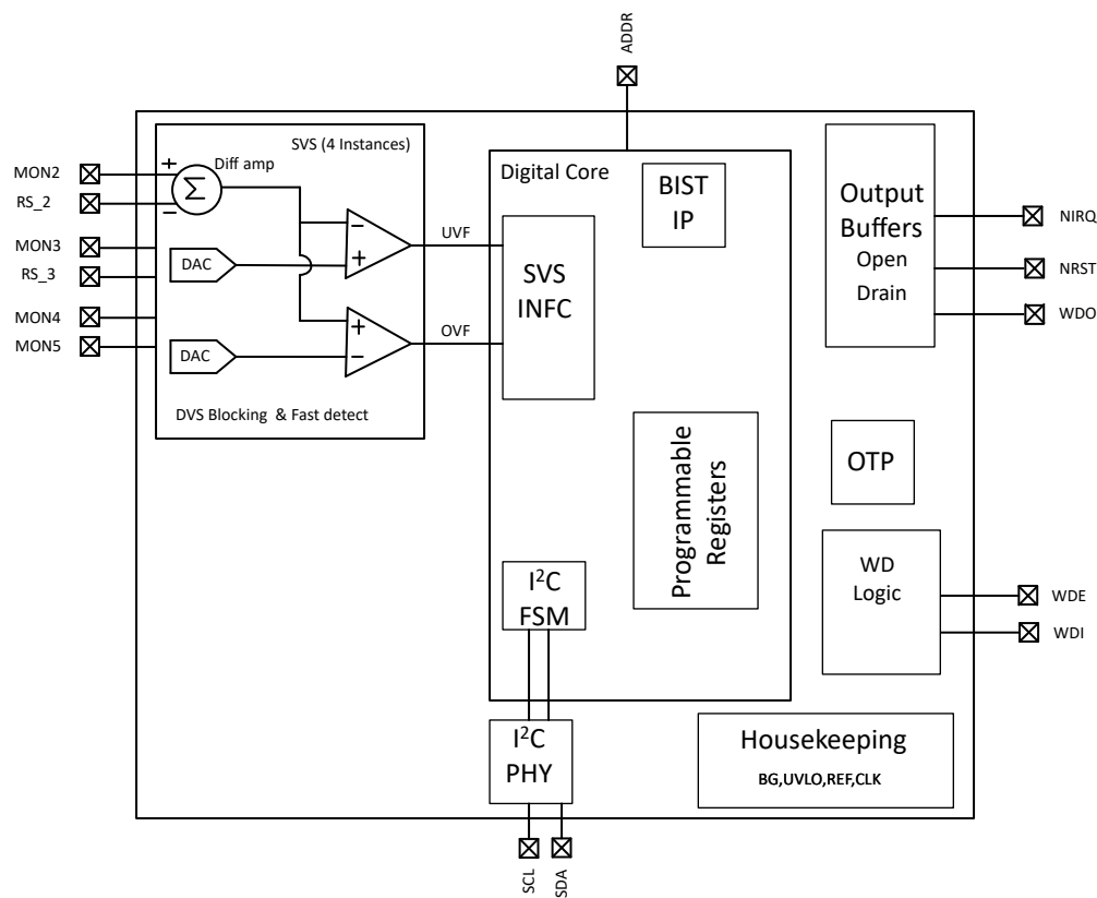
图 7-1. TPS388C04-Q1 方框图
