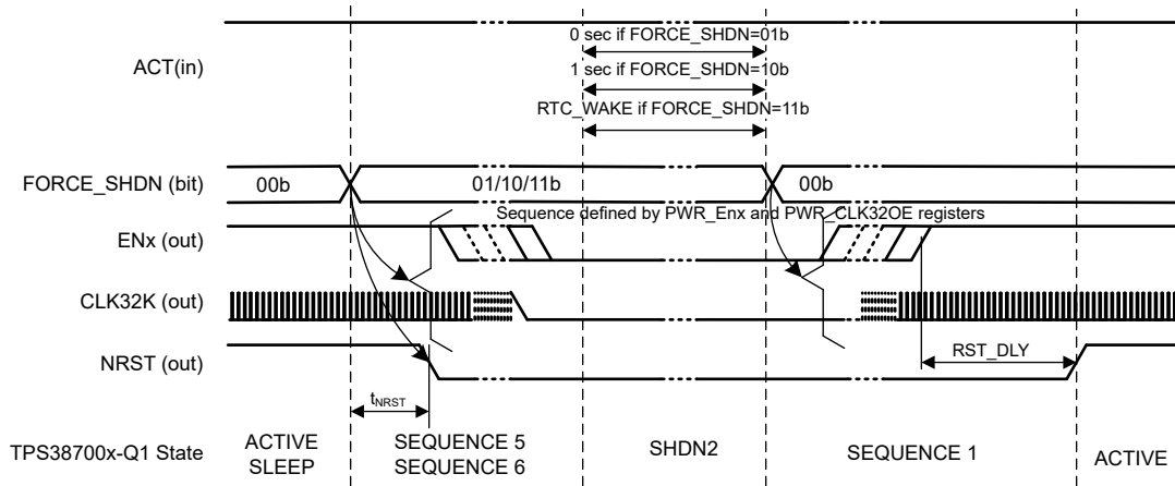
图 7-6. 从 SHDN2 上电 - 在 FORCE_SHDN ≠ 00b 的情况下关闭软件
