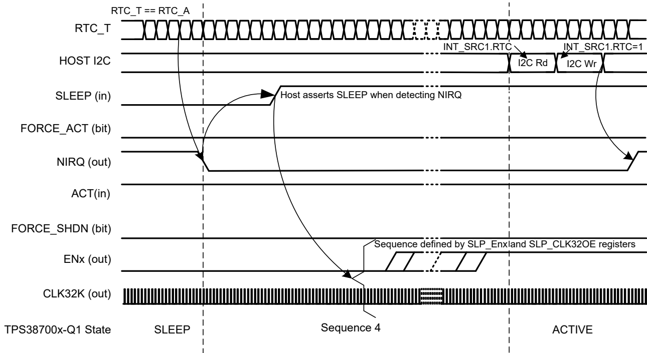
图 7-10. 已触发睡眠退出 RTC - \overline{\text{SLEEP}} 时序
