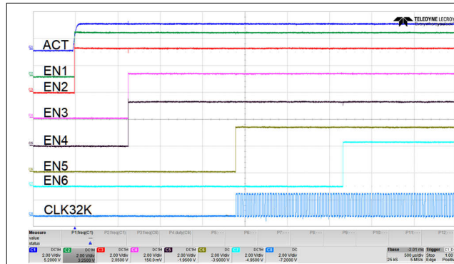
图 8-2. 上电序列
