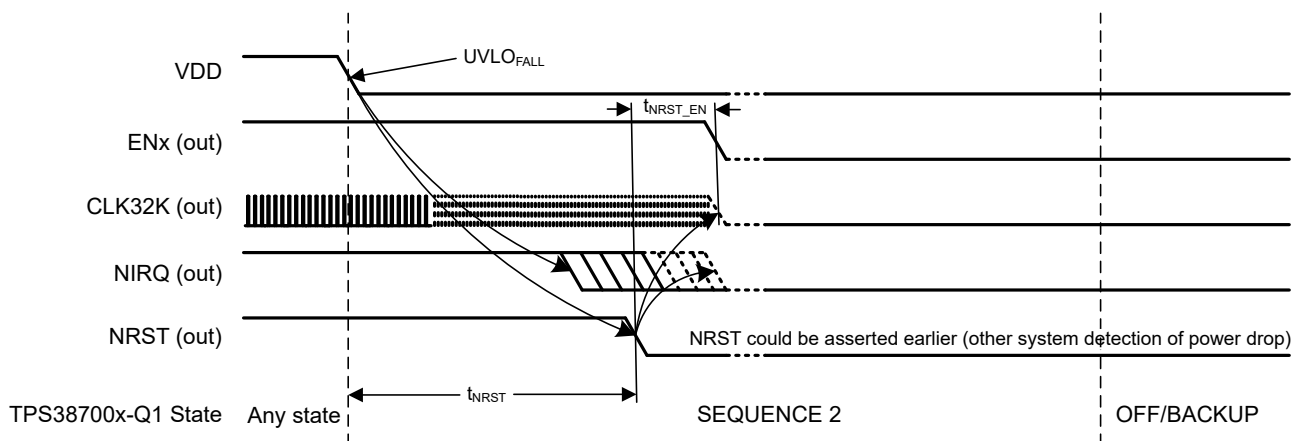
图 7-7. 紧急断电
