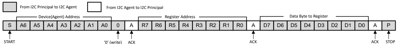
图 7-17. I2C 单字节写入
