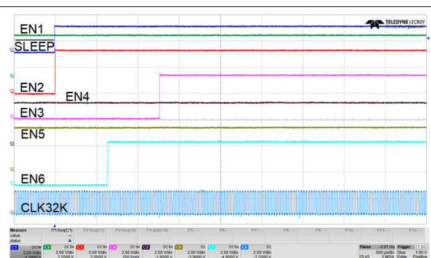
图 8-5. 睡眠退出序列
