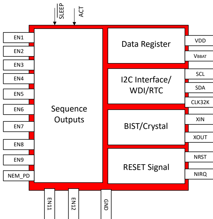
图 7-1. TPS38700-Q1 方框图
