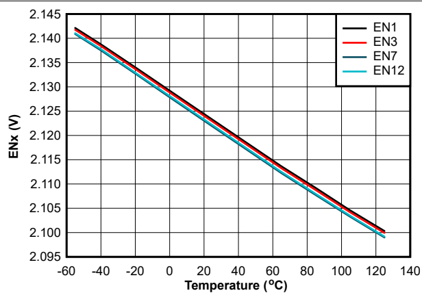
图 6-8. ENx 逻辑高电平输出电压与温度间的关系
