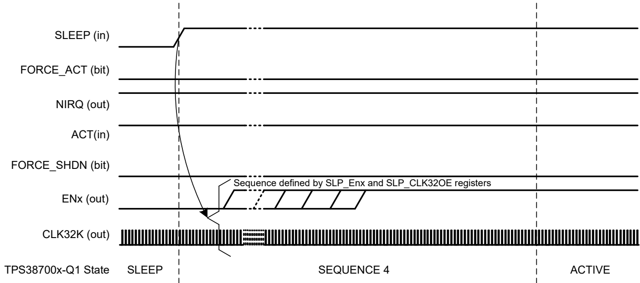
图 7-9. 已触发睡眠退出 \overline{\text{SLEEP}}
