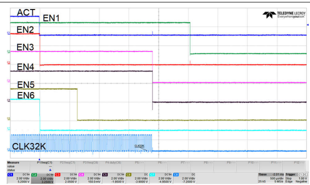
图 8-3. 断电序列
