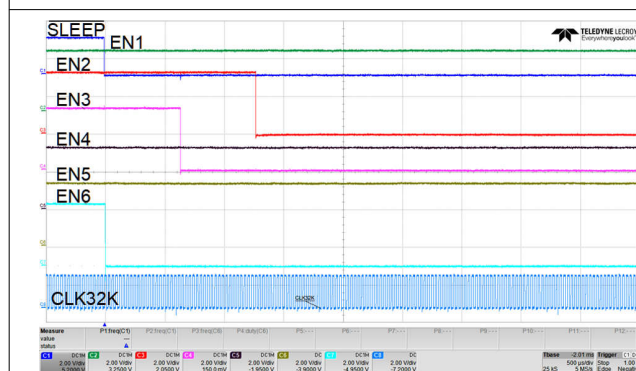
图 8-4. 睡眠进入序列
