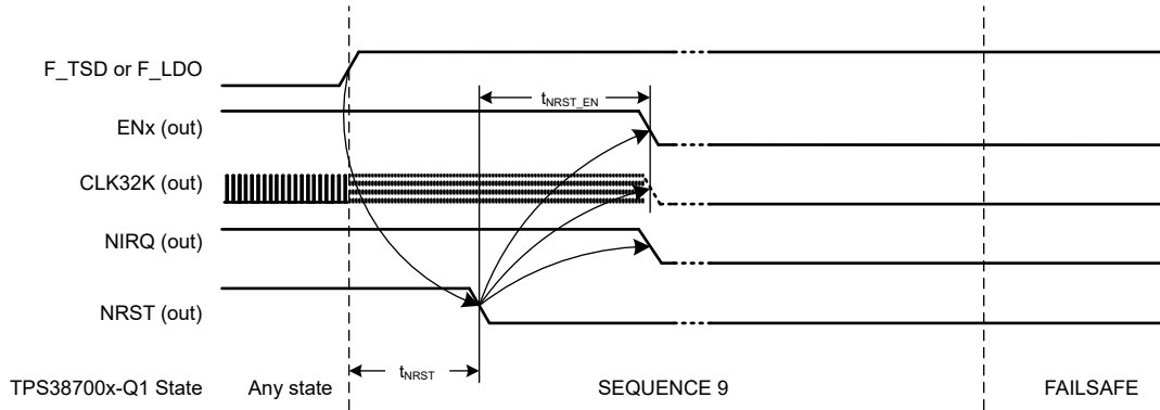
图 7-15. 失效防护断电
