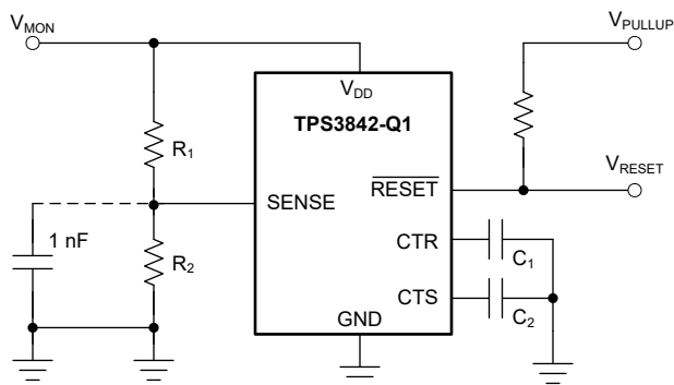
图 7-3. 使用 TPS3842A011DRLRQ1 监控用户定义的阈值电压
