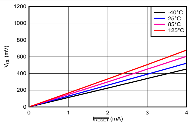
图 6-7. RESET 灌电流与 V_{\text{OL}} 间的关系 ( V_{DD} = 3.3\text{V} )
