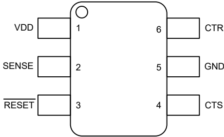
图 5-1. DRL 封装 6 引脚 SOT5X3 顶视图
