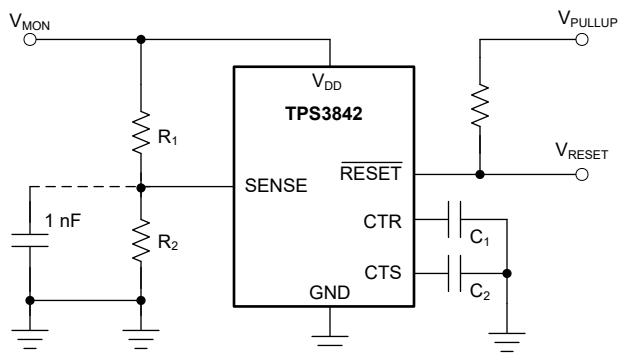
图 7-3. 使用 TPS3842A011DR1R 监控用户定义的阈值电压
