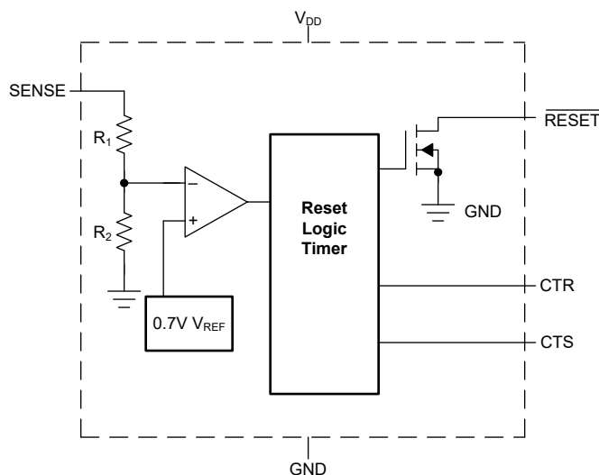
图 7-2. 固定电压版本
