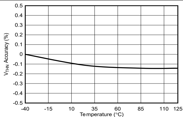
图 6-3. V_{\text{THN}} 精度与温度间的关系
