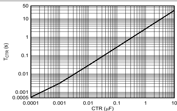
图 6-4. T_{\text{CTR}} 与 \text{CTR} 间的关系
