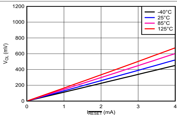
图 6-8. RESET 灌电流与 V_{\text{OL}} 间的关系 ( V_{\text{DD}} = 12\text{V} )
