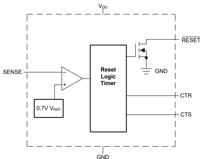
图 7-1. 可调电压版本
