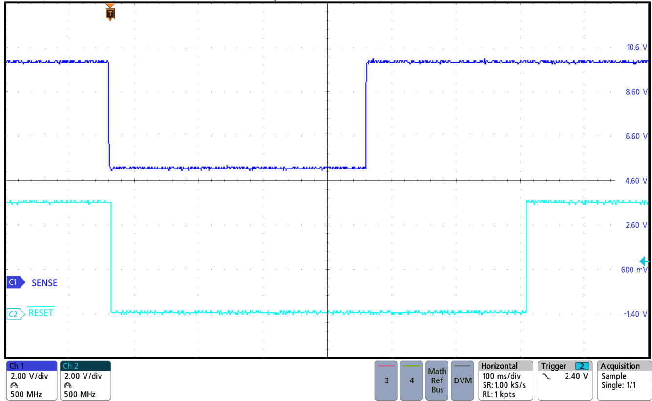
图 8-2. TPS3842 检测欠压故障和 RESET 恢复
