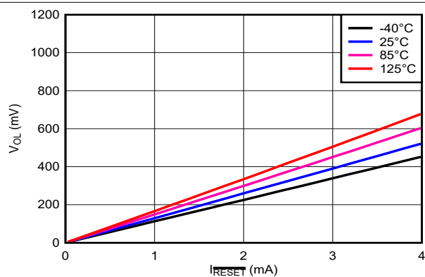
图 6-7. RESET 灌电流与 V_{\text{OL}} 间的关系 ( V_{\text{DD}} = 3.3\text{V} )
