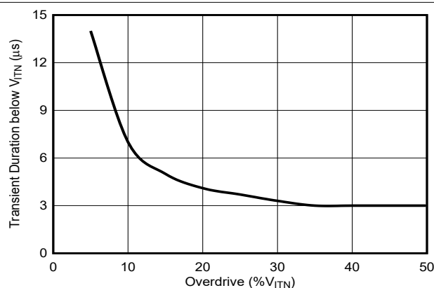
图 6-6. SENSE 上的瞬态持续时间与 SENSE 阈值过驱电压间的关系 (CTS = 开路)
