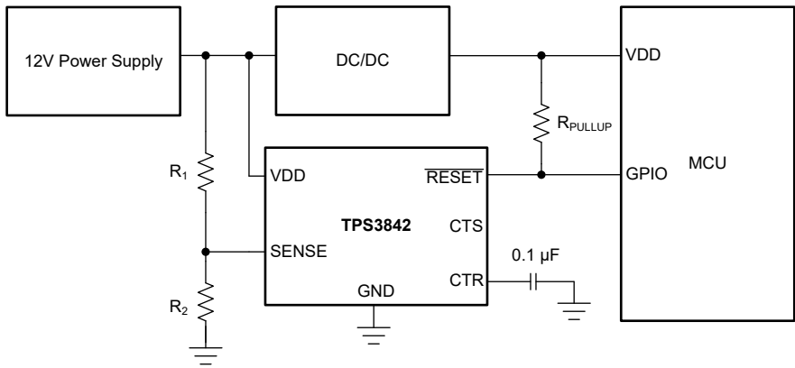
图 8-1. 使用 TPS3842 监控 12V 电源的典型应用
