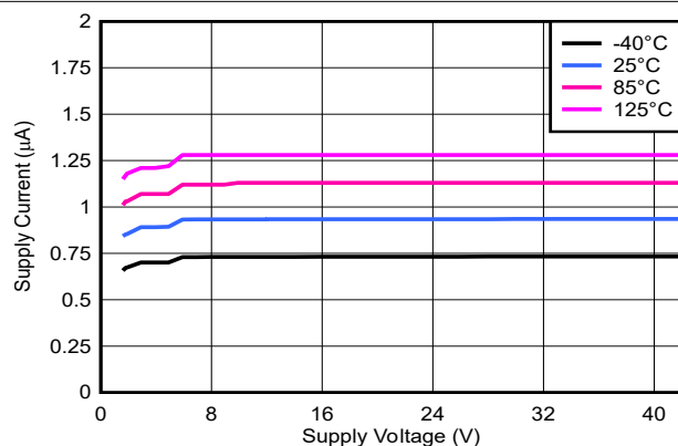
图 6-2. 电源电流与电源电压间的关系
