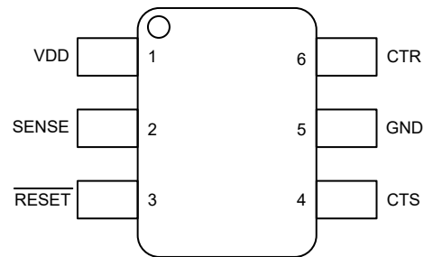
图 5-1. DRL 封装 6 引脚 SOT5X3 顶视图
