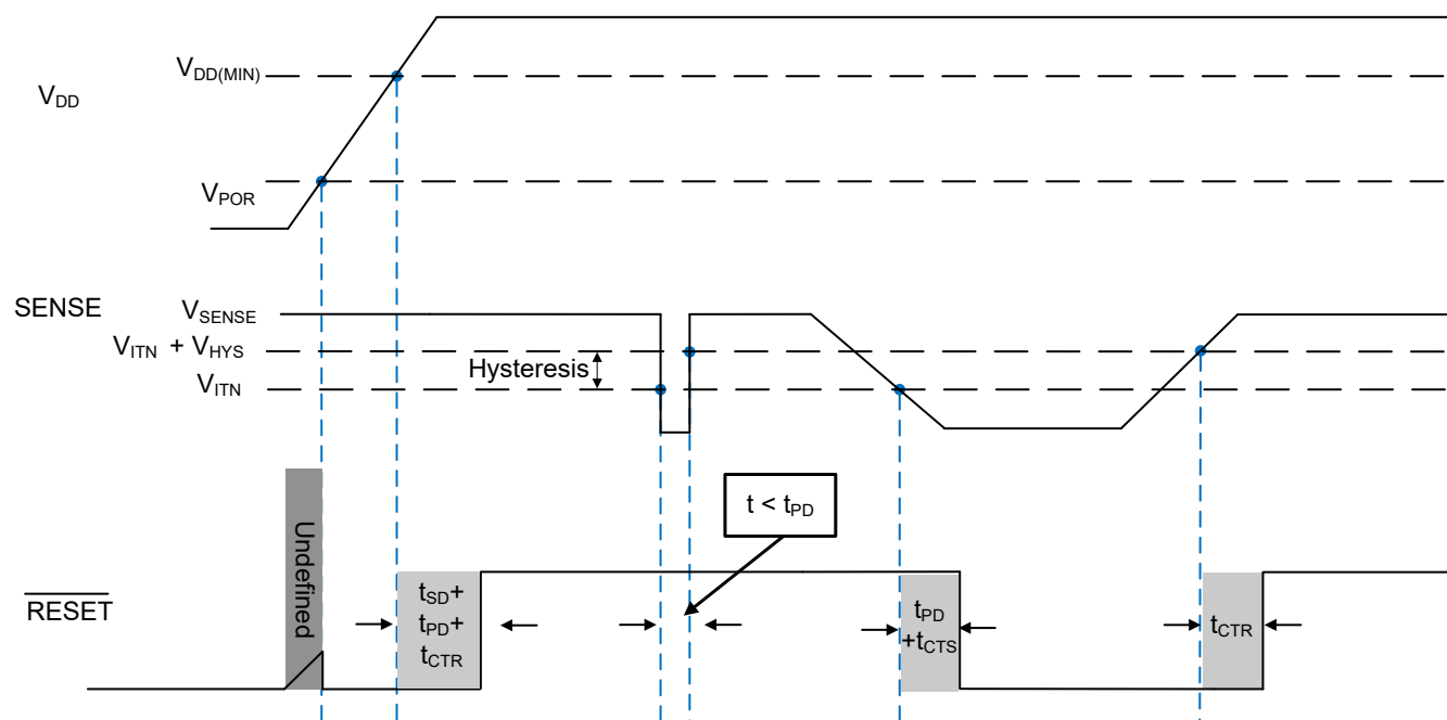
图 6-1. 时序图
