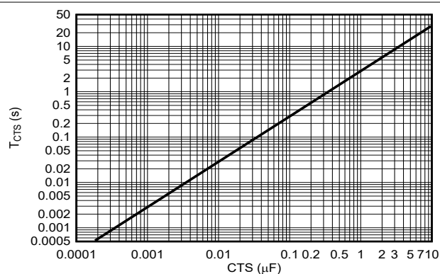
图 6-5. T_{\text{CTS}} 与 \text{CTS} 间的关系
