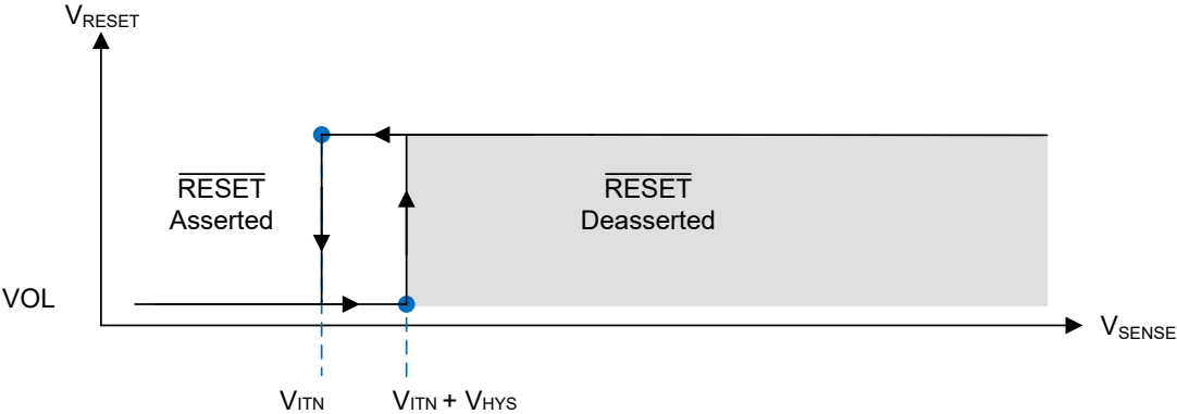
图 7-4. 迟滞 ( 欠压低电平有效 )
