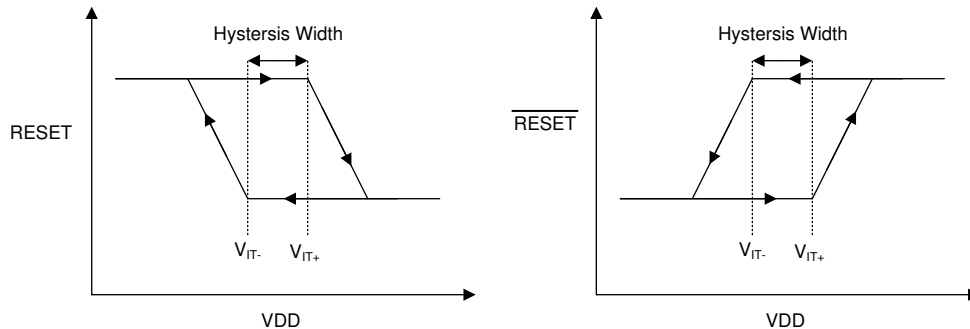
图 44. Hysteresis Diagram
