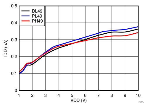
TPS3840 典型电源电流
