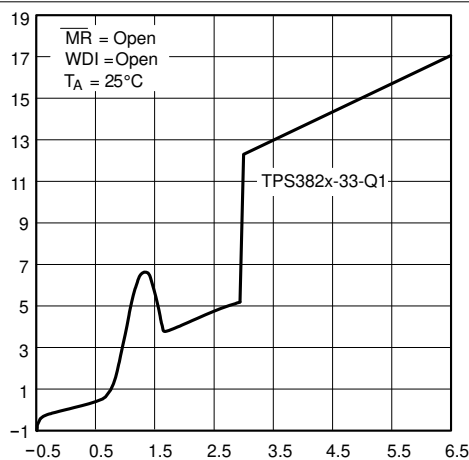
图 6-3. 电源电流与电源电压间的关系
