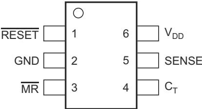
图 5-1. DBV 封装 6 引脚 SOT-23 顶视图
