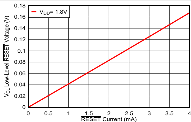
图 7-6. 低电平 \overline{\text{RESET}} 电压与 \overline{\text{RESET}} 电流间的关系
