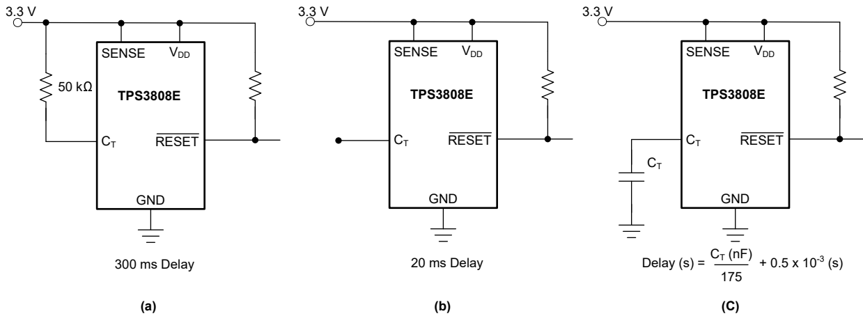
图 8-4. 用于设置 \overline{RESET} 延迟时间的配置
