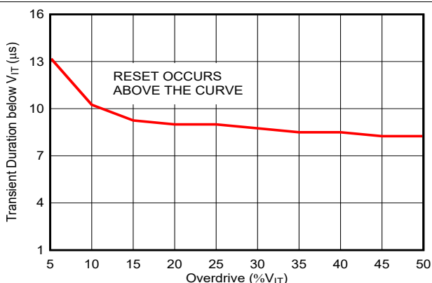
图 7-4. \text{SENSE} 上的最大瞬态持续时间与 \text{SENSE} 阈值过驱电压间的关系
