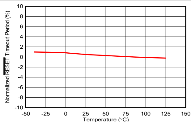
图 7-3. 标准化 \overline{\text{RESET}} 超时周期与温度间的关系 ( C_T = \text{开路} , C_T = V_{DD} , C_T = \text{任意} )
