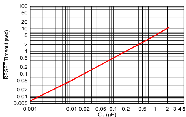
图 7-2. \overline{\text{RESET}} 超时周期与 C_T 间的关系
