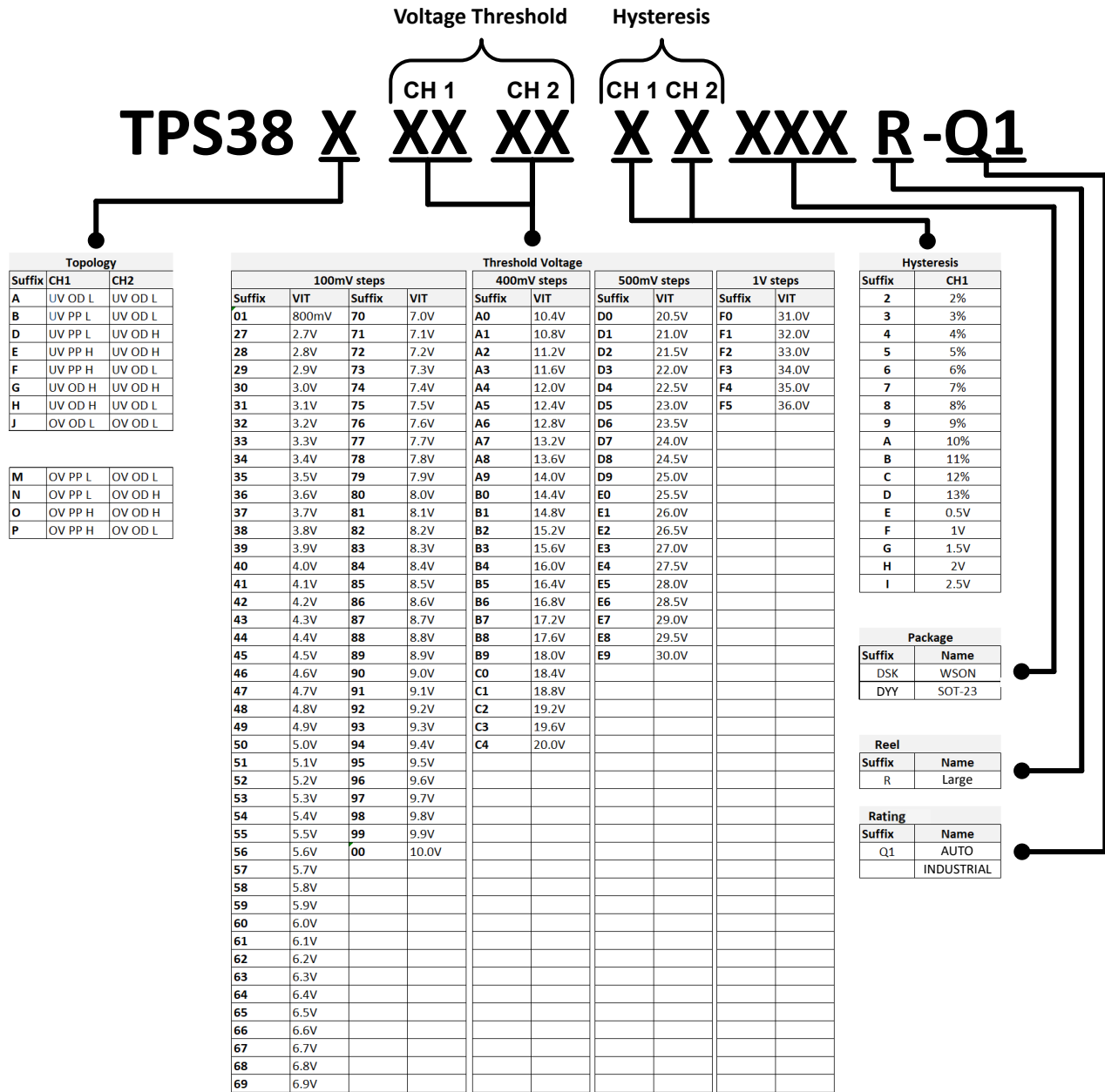
图 5-1. Device Nomenclature
