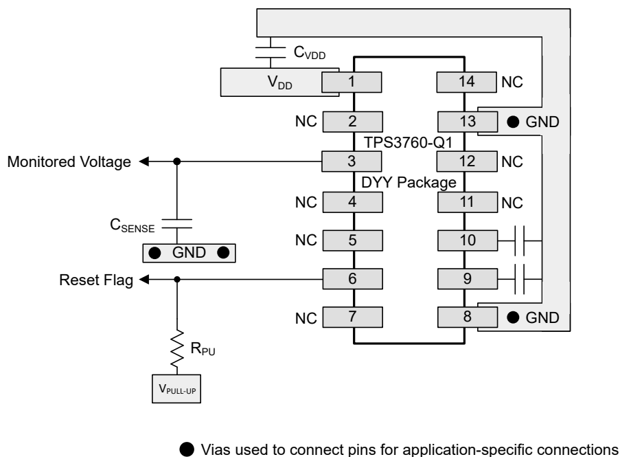
图 9-5. TPS3760-Q1 Recommended Layout
