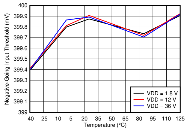
典型误差与结温之间的关系
