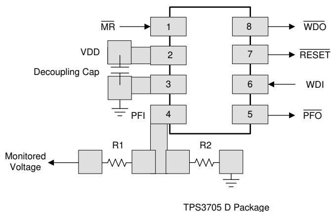
图 11-1. TPS3705 Layout
