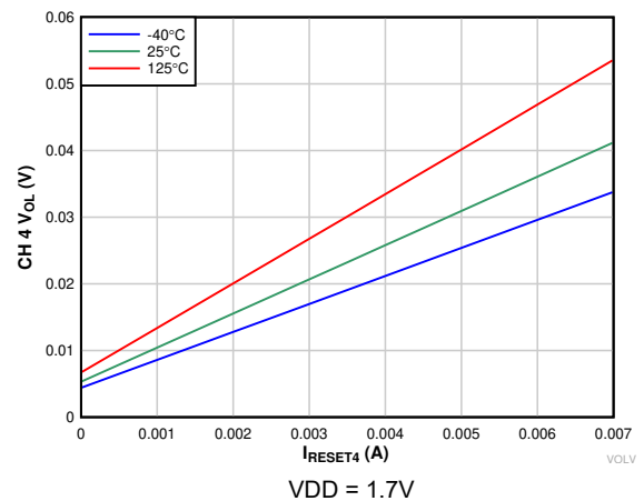
图 6-14. 低电平 CH 4 输出电压与 RESET4 电流间的关系
