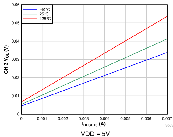
图 6-13. 低电平 CH 3 输出电压与 RESET3 电流间的关系
