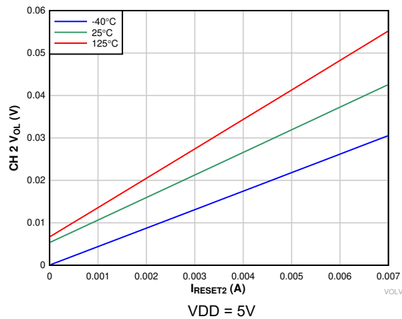
图 6-11. 低电平 CH 2 输出电压与 RESET2 电流间的关系
