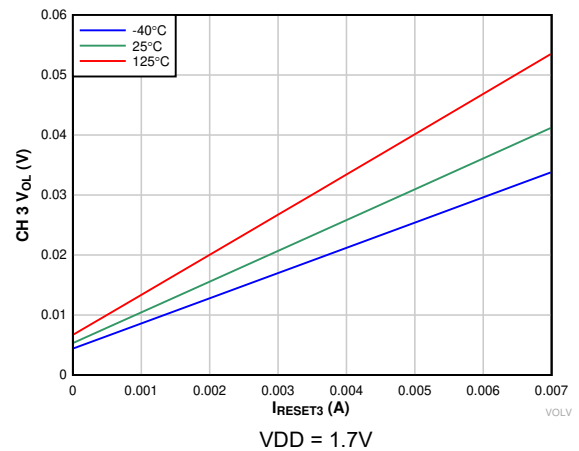
图 6-12. 低电平 CH 3 输出电压与 RESET3 电流间的关系
