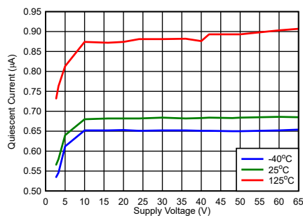
典型 I_{DD} 与 V_{DD}
