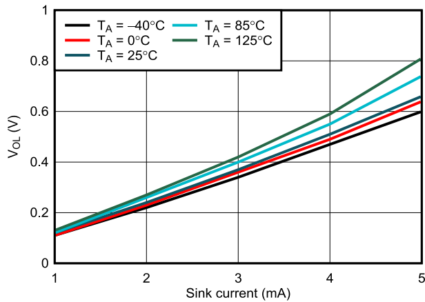
图 6-10. RESET V_{OL} 与 I_{sink} 间的关系, V_{DD} = 1.5V
