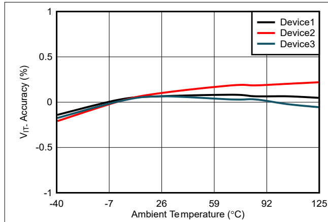
图 6-2. V_{IT} 精度与温度间的关系
