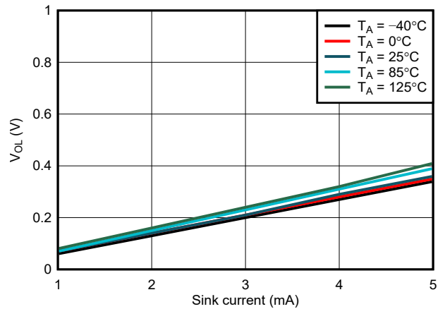
图 6-11. WDO V_{OL} 与 I_{sink} 间的关系, V_{DD} = 1.5V
