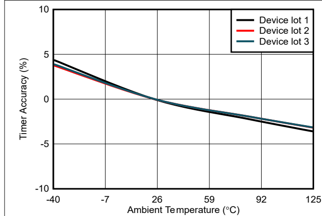
图 6-6. 计时器精度与温度间的关系
