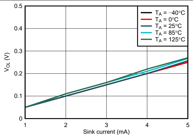
图 6-13. WDO V_{OL} 与 I_{sink} 间的关系, V_{DD} = 3.3V
