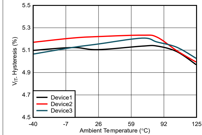
图 6-4. V_{IT} 迟滞与温度间的关系
