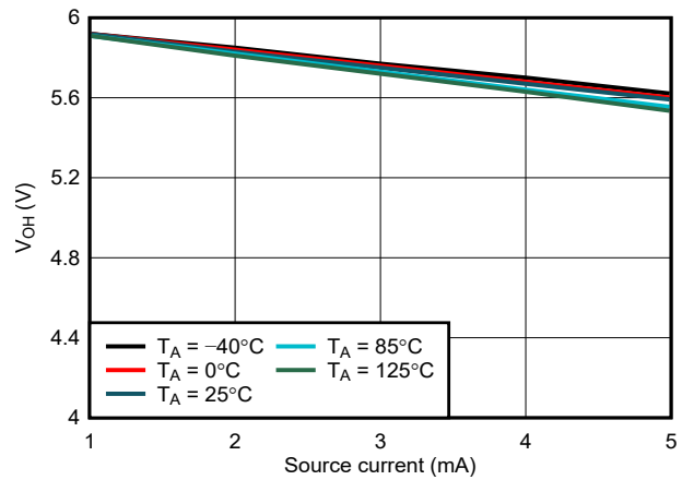
图 6-17. WDO V_{OH} 与 I_{source} 间的关系, V_{DD} = 6.0V
