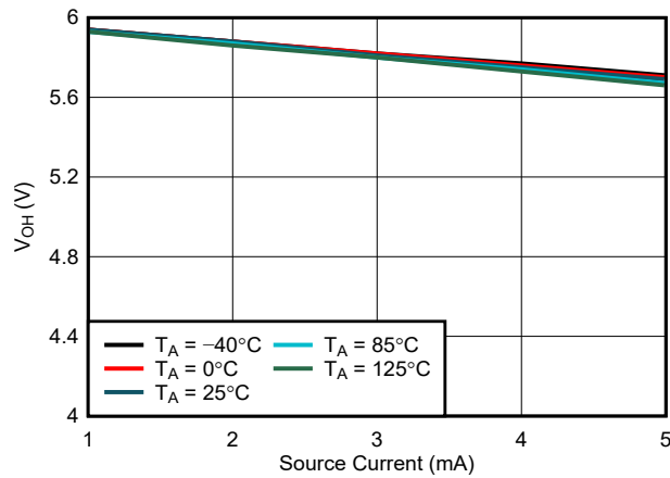
图 6-16. RESET V_{OH} 与 I_{source} 间的关系, V_{DD} = 6.0V
