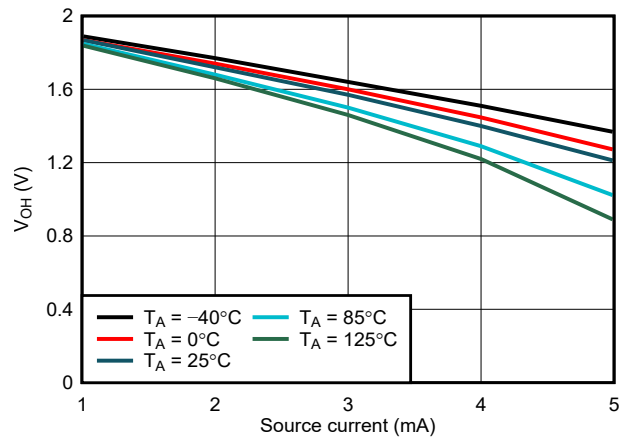
图 6-15. WDO V_{OH} 与 I_{source} 间的关系, V_{DD} = 2.0V
