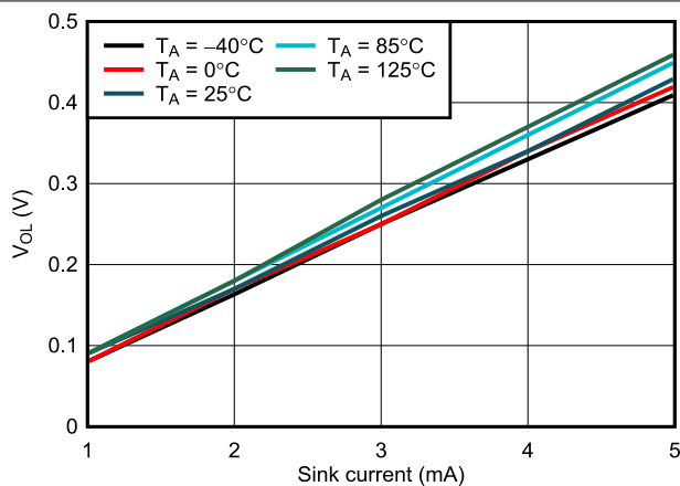
图 6-12. RESET V_{OL} 与 I_{sink} 间的关系, V_{DD} = 3.3V
