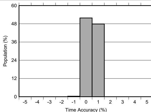
图 7-3. 计时器精度直方图
