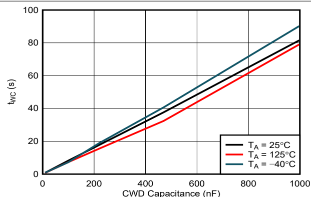
图 7-4. t_{WC} 与电容间的关系
