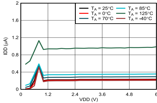
图 7-10. 电源电流与电源电压间的关系
