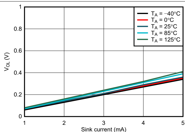
图 7-6. WDO V_{OL} 与 I_{sink} 间的关系, V_{DD} = 1.5\text{V}
