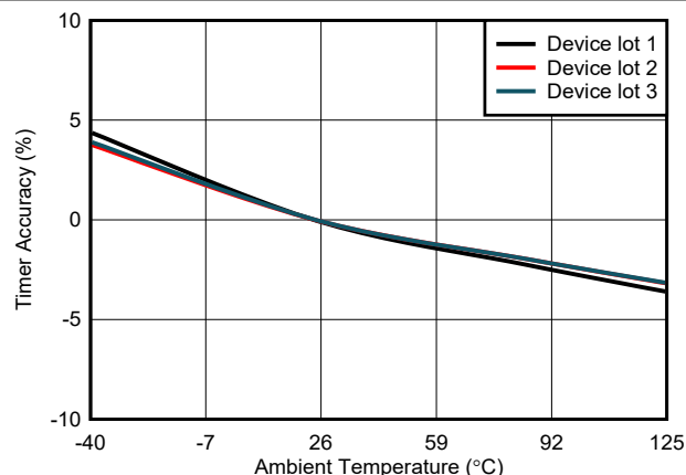
图 7-2. 计时器精度与温度间的关系
