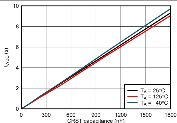
图 7-5. t_{WDO} 与电容间的关系
