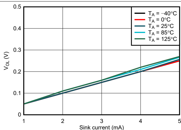
图 7-7. WDO V_{OL} 与 I_{sink} 间的关系, V_{DD} = 3.3\text{V}
