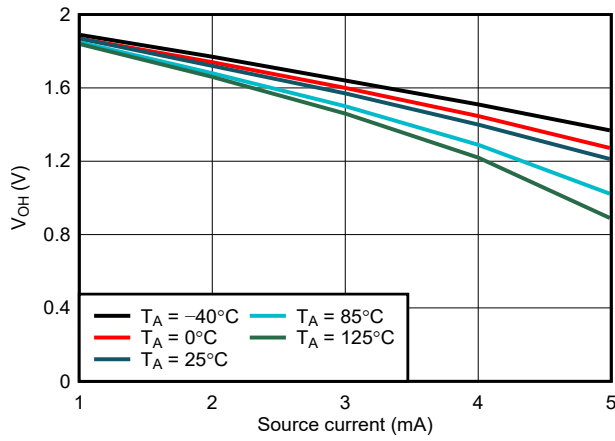
图 7-8. WDO V_{OH} 与 I_{source} 间的关系, V_{DD} = 2.0\text{V}
