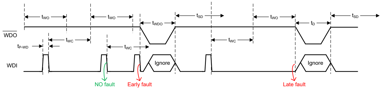
图 8-4. 窗口看门狗计时器运行情况
