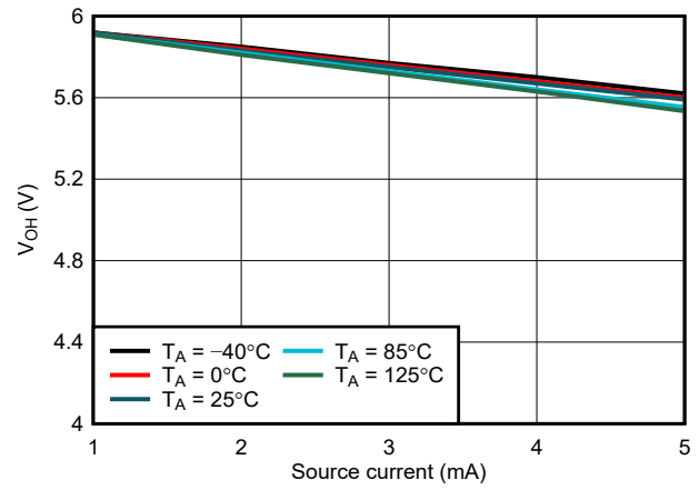
图 7-9. WDO V_{OH} 与 I_{source} 间的关系, V_{DD} = 6.0\text{V}
