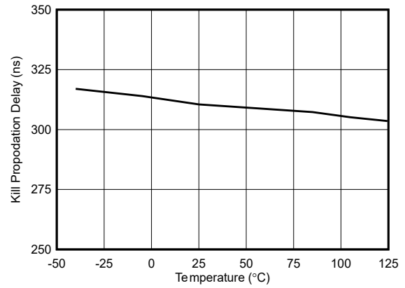
图 6-12. KILL 传播延迟与温度间的关系
