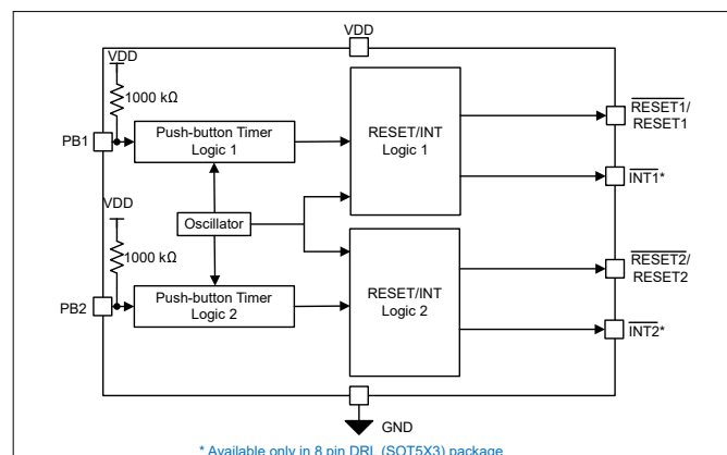
图 7-1. TPS3423 方框图 (低电平有效按钮输入)
