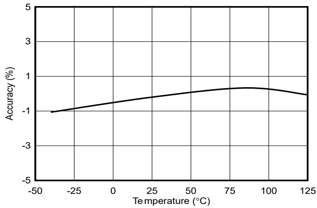
图 6-11. 计时精度与温度间的关系 (短按、长按、KILL 消隐时间)
