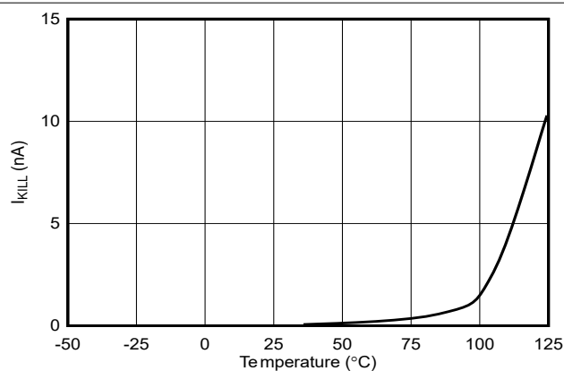
图 6-8. KILL 电流与温度间的关系
