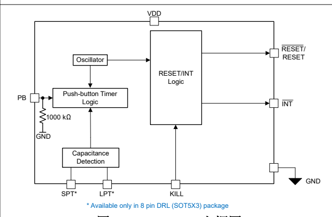
图 7-4. TPS3424 方框图 (高电平有效按钮输入)
