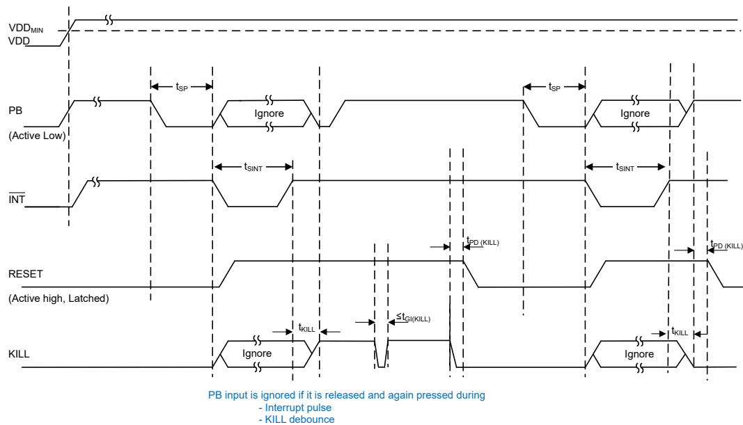
图 6-4. 时序图：KILL
