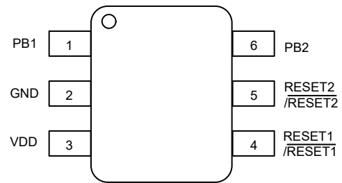
图 5-2. 引脚配置选项 TPS3423 DRL 封装 6 引脚 SOT-5X3 顶视图
