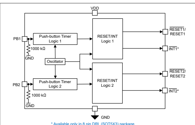
图 7-2. TPS3423 方框图 (高电平有效按钮输入)
