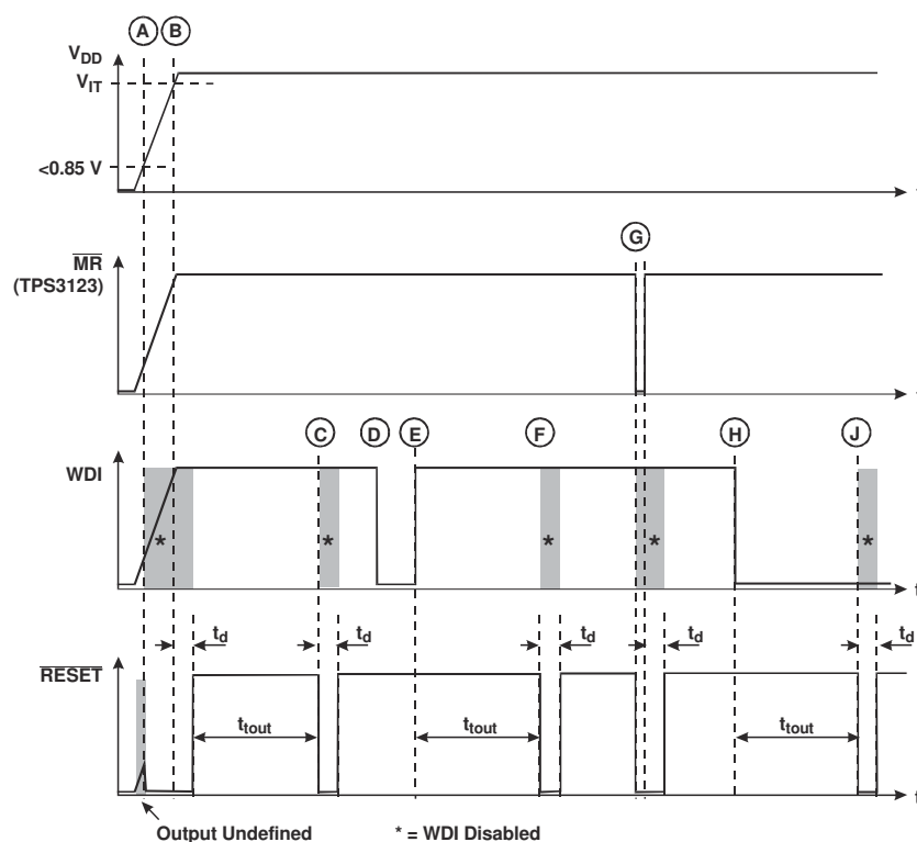
图 6-2. 时序图 TPS3123/4/8
