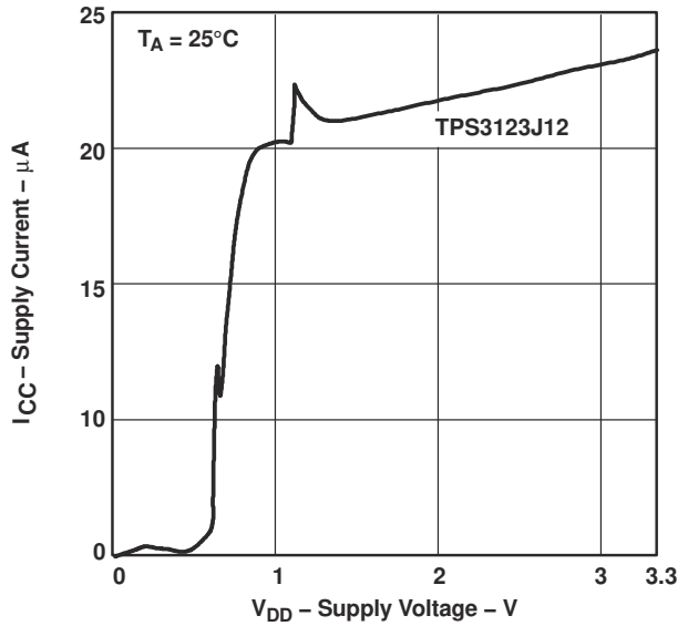
图 6-3. 电源电流与电源电压间的关系
