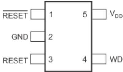
图 5-2. TPS3124 : DBV 封装 5 引脚 SOT-23 顶视图
