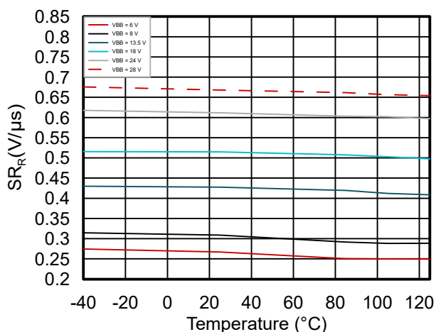
图 6-12. 在 V_{BB} 电压范围内 SR_R 与温度间的关系
