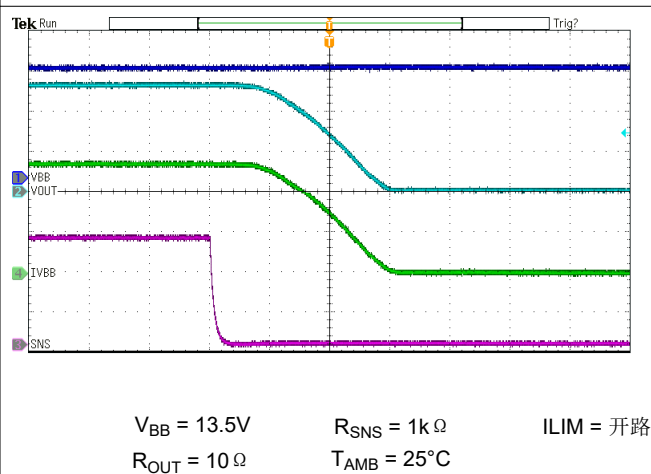
图 6-14. 开关关断
