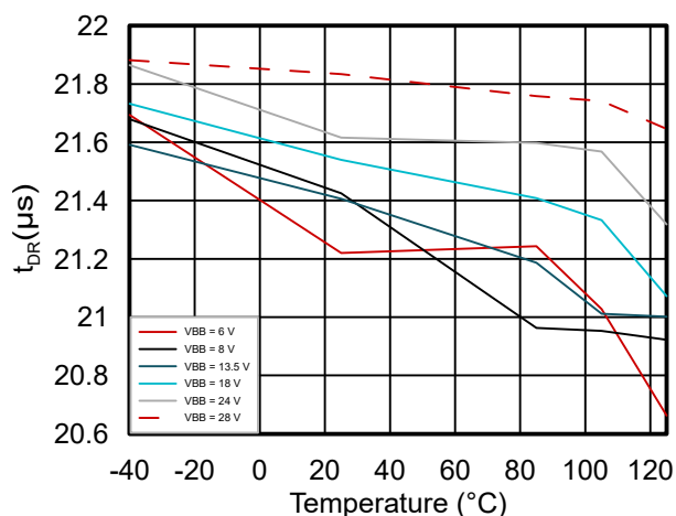
图 6-11. 在 V_{BB} 电压范围内 T_{DR} 与温度间的关系
