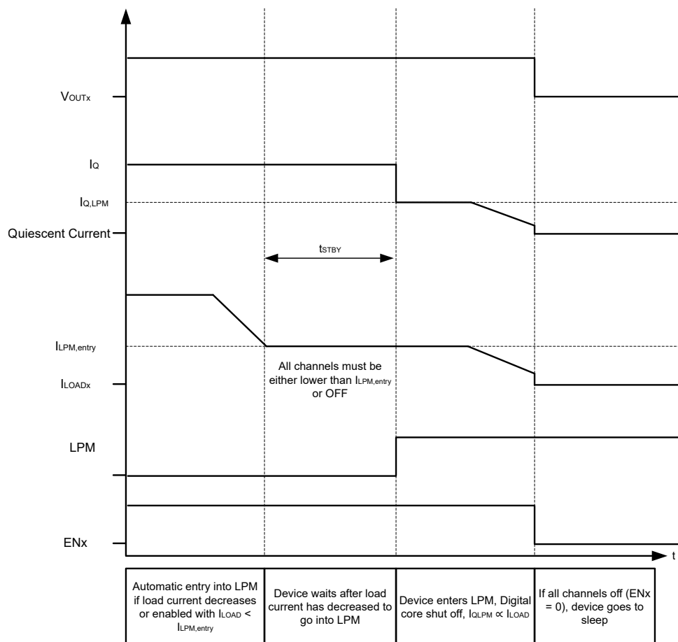
图 7-2. 进入 LPM
