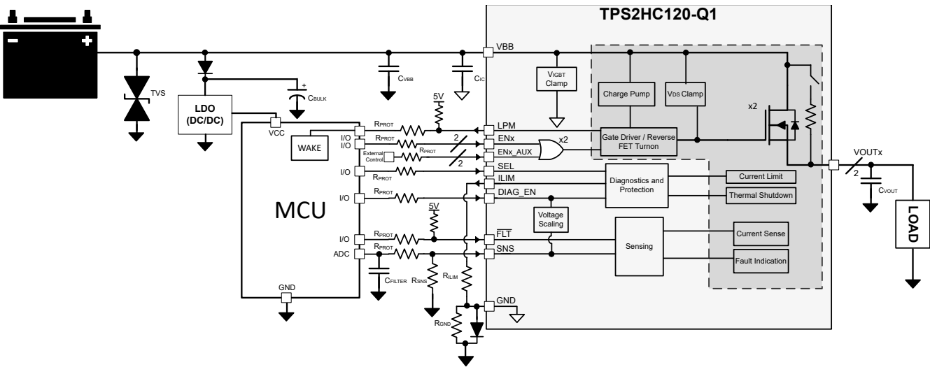
图 8-1. 典型应用图
