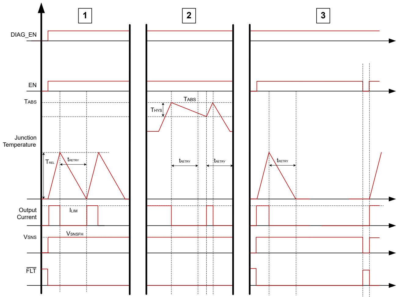
图 7-17. 热行为
