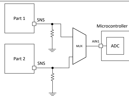
图 7-14. 跨多个器件共享 SNS 方法 2
