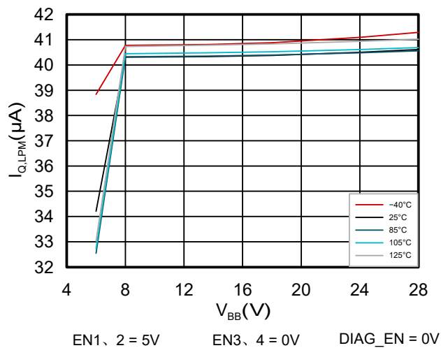
图 6-7. 启用 2 个通道时, 不同温度条件下 I_{Q,LPM} 与 V_{BB} 间的关系
