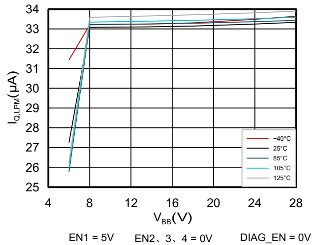
图 6-6. 启用 1 个通道时, 不同温度条件下 I_{Q,LPM} 与 V_{BB} 间的关系
