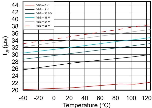
图 6-9. 在 V_{BB} 电压范围内 T_{DF} 与温度间的关系
