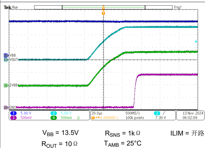
图 6-13. 开关导通
