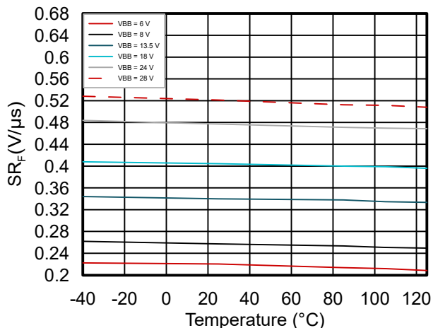
图 6-10. 在 V_{BB} 电压范围内 SR_F 与温度间的关系
