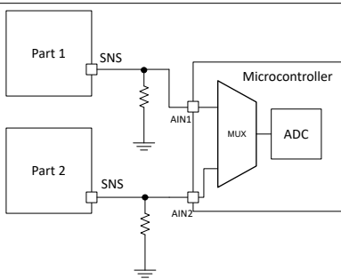
图 7-13. 跨多个器件共享 SNS 方法 1
