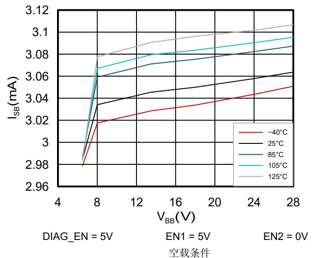
图 6-8. 不同温度条件下 I_{SB} 与 V_{BB} 间的关系
