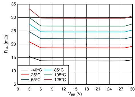
图 10. On Resistance ( R_{ON} ) vs V_{BB}
