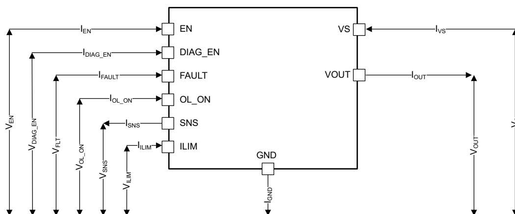
图 7-1. 参数定义
