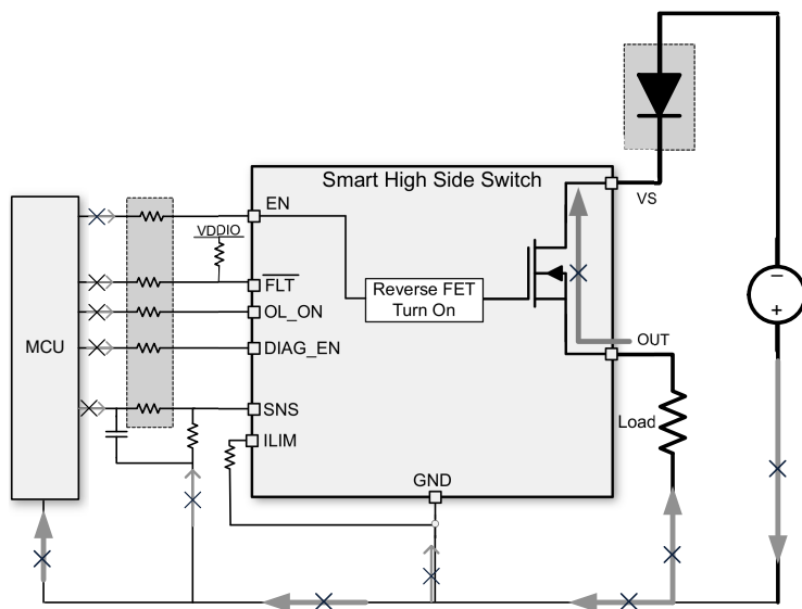
图 8-17. 采用阻断二极管实现反向保护
