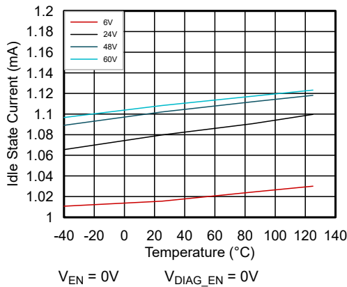
图 6-3. 来自 VS 输入电源的空闲状态电流 ( I_{IDLE,vs} ) 与温度与 VS 电压间的关系 V_{EN} = 0V V_{DIAG\_EN} = 0V
