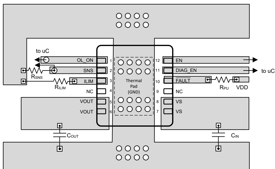
图 9-4. 不采用接地网络的 DNT 布局
