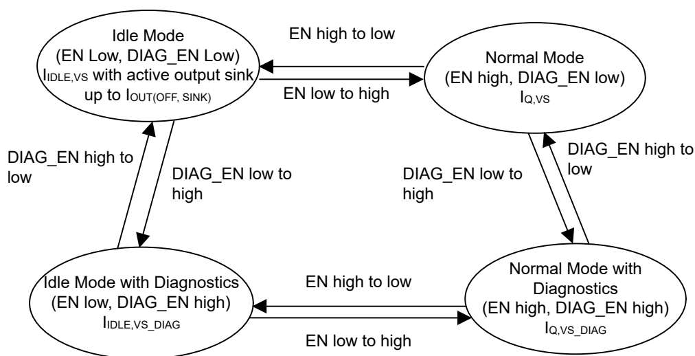
图 8-1. 工作模式状态机
