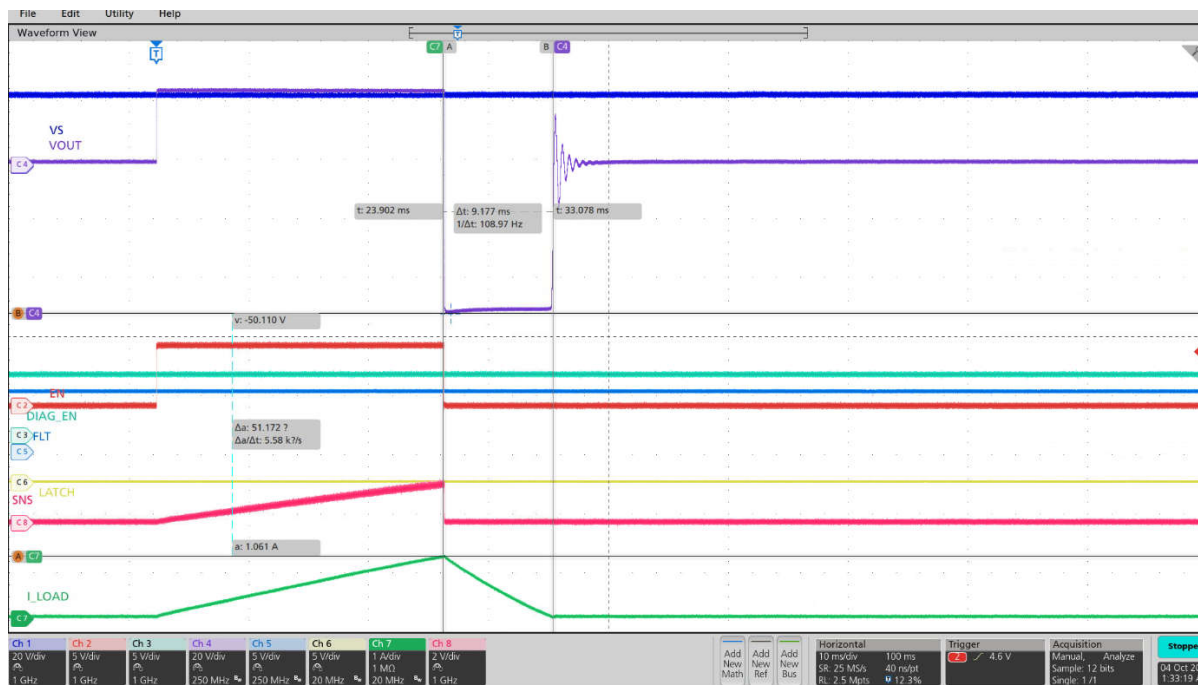
图 8-13. TPS281C100 电感放电 (400mH)
