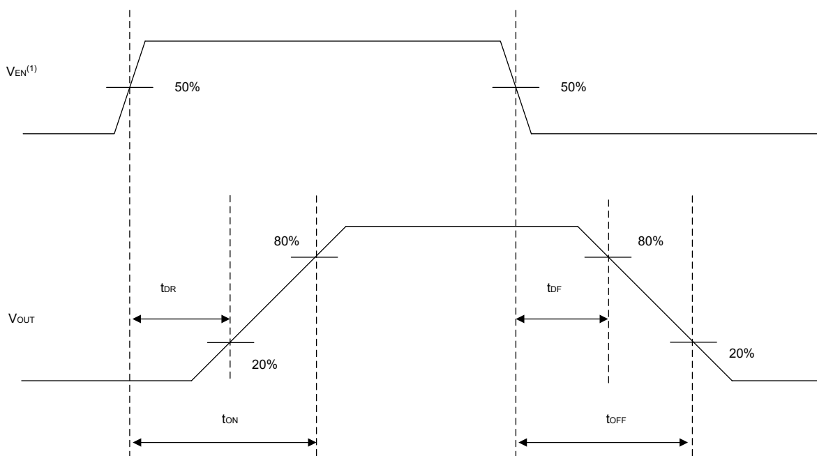
图 7-1. 参数定义
