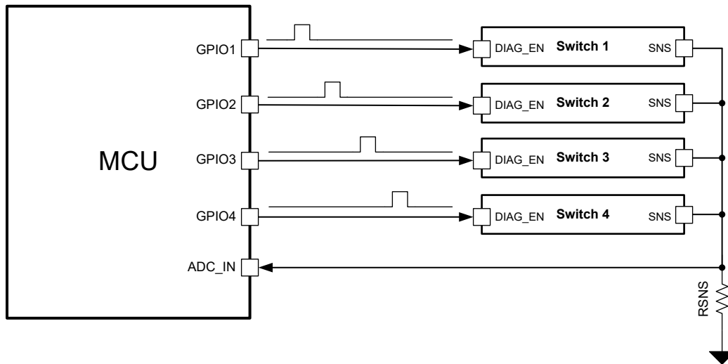
图 8-20. 电阻器共享
