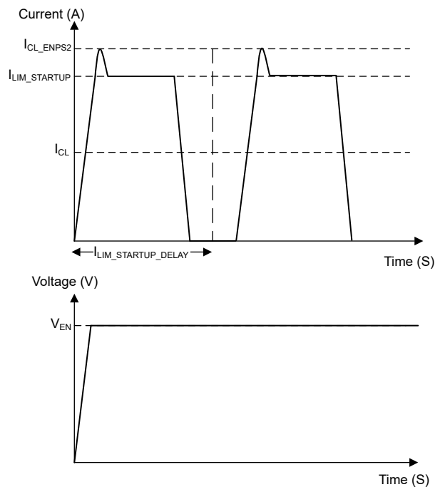
图 8-10. ILIM_STARTUP_DELAY 之后的自动重试行为
