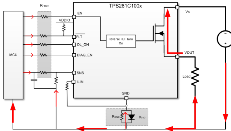
图 8-18. 通过接地网络实现反向保护
