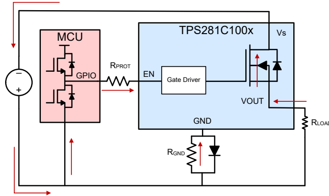
图 8-19. MCU IO 保护
