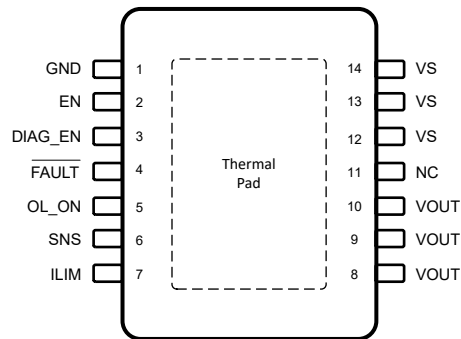
图 5-1. PWP 引脚，14 引脚 HTSSOP（顶视图）
