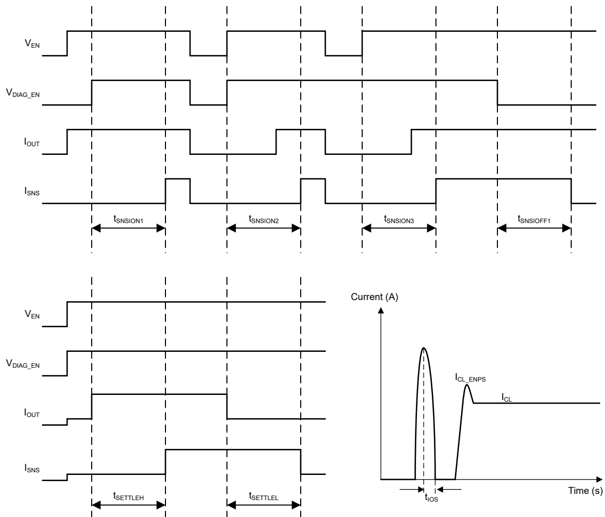
图 7-3. SNS 时序特性定义
