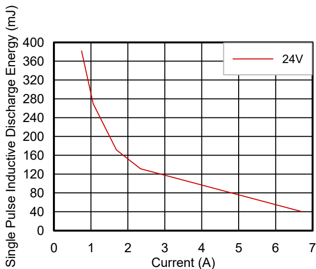
图 8-14. TPS281C100 在 125°C 和 24V 电源条件下的电感负载放电能量能力
