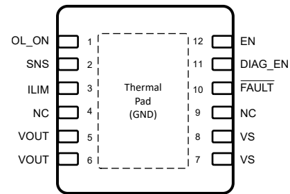
图 5-2. DNT 封装，12 引脚 WSON（顶视图）
