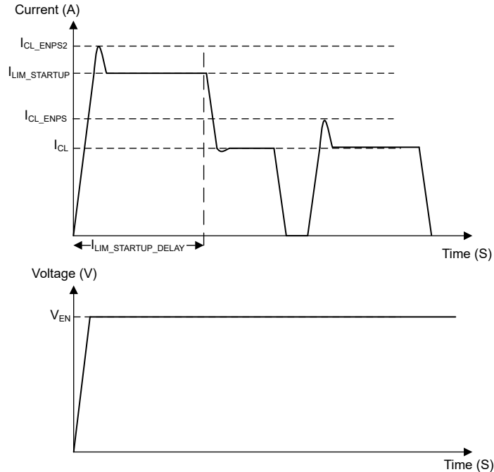
图 8-9. ILIM_STARTUP_DELAY 之前的自动重试行为
