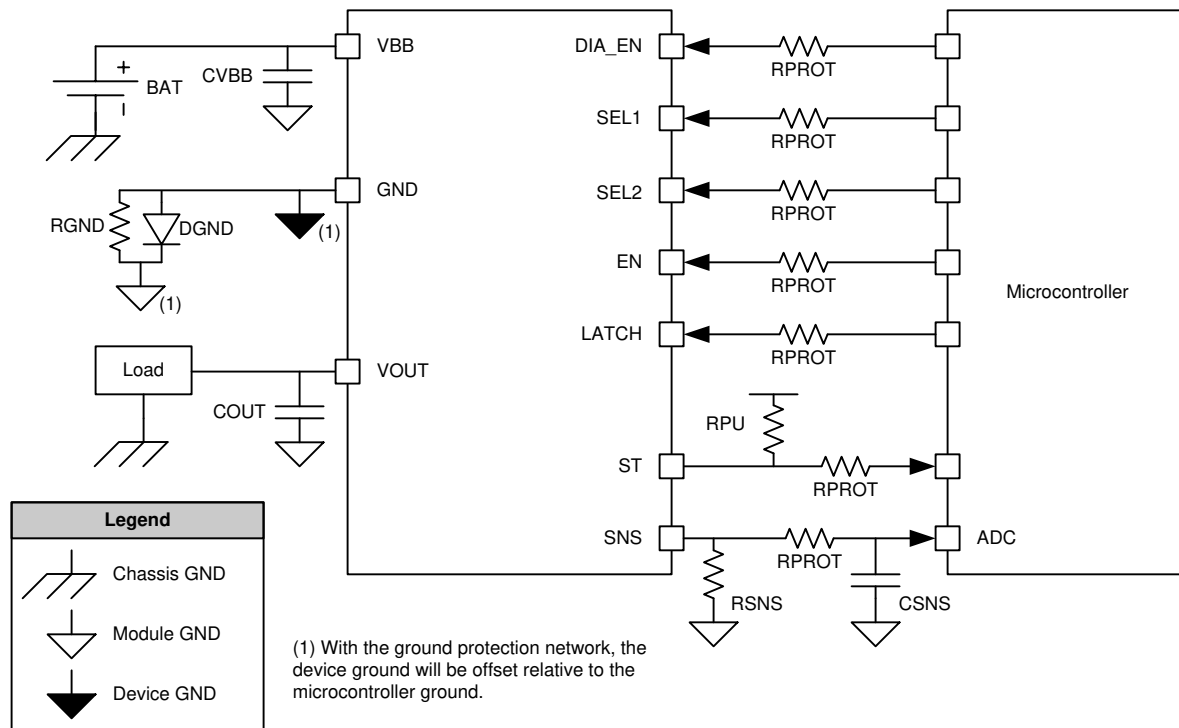
图 10-1. System Diagram
