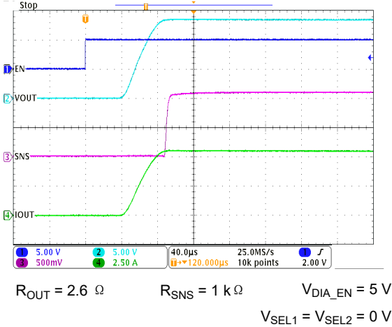
图 7-27. Turn-on Time ( t_{ON} )
