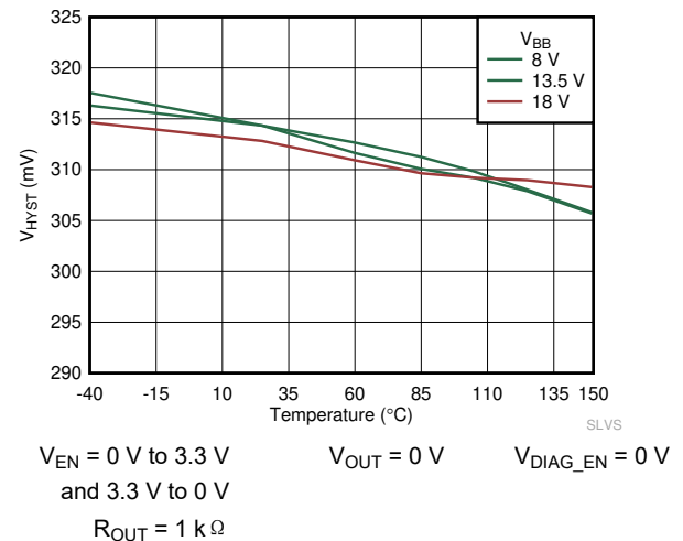
图 7-24. V_{IHYS} vs Temperature
