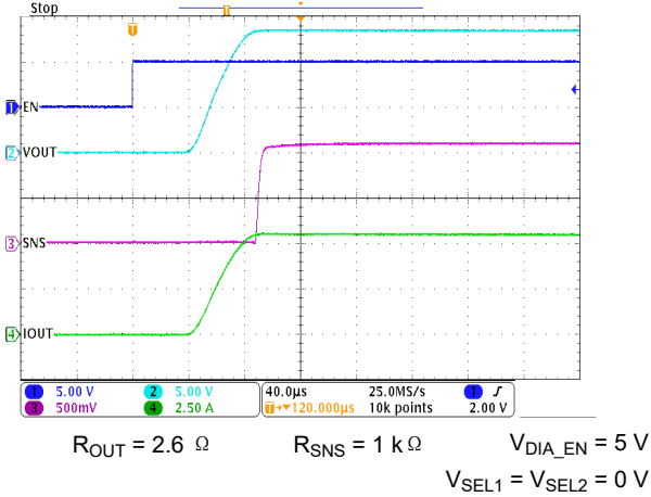
图 7-27. Turn-on Time ( t_{ON} )
