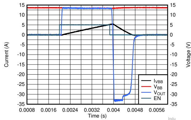
图 7-33. Inductive Load Demagnetization
