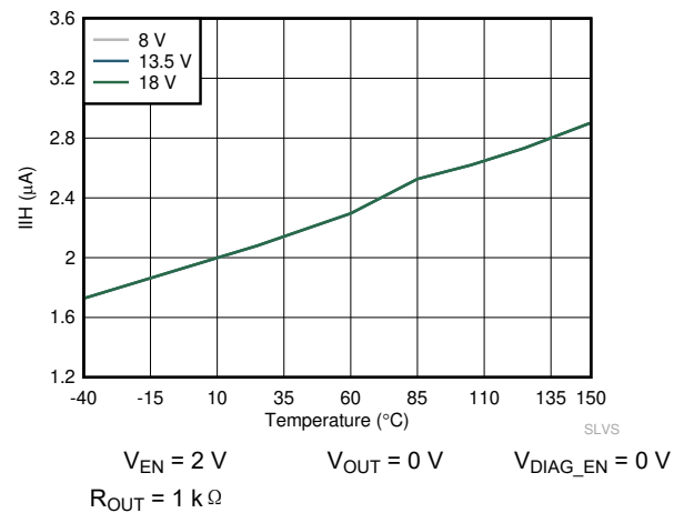
图 7-26. I_{IH} vs Temperature
